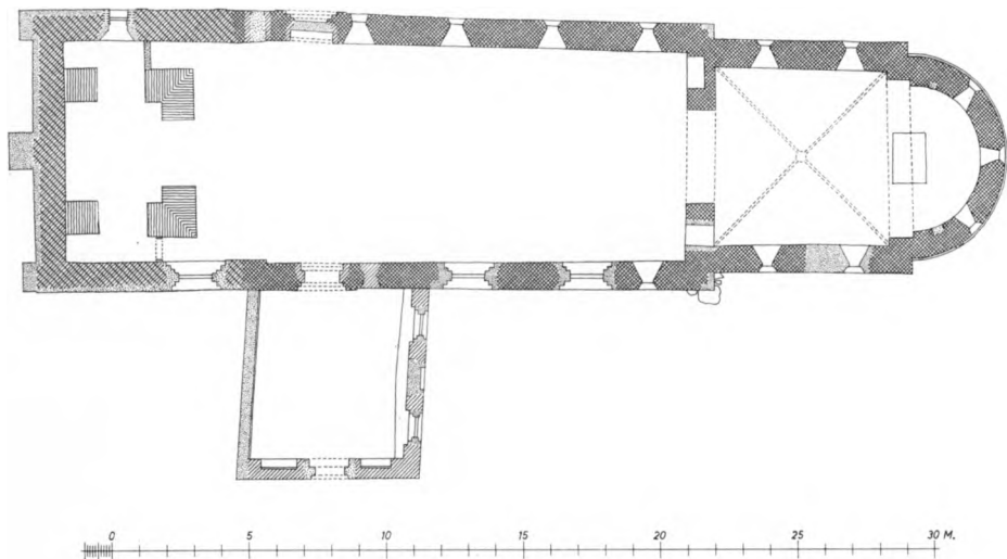
Fig. 2. Bylderup. Plan. 1:300. Målt af El. M. 1954.
