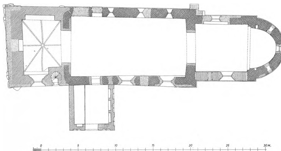
Fig. 2. Tinglev. Plan. 1:300. Målt af El. M. 1956.
