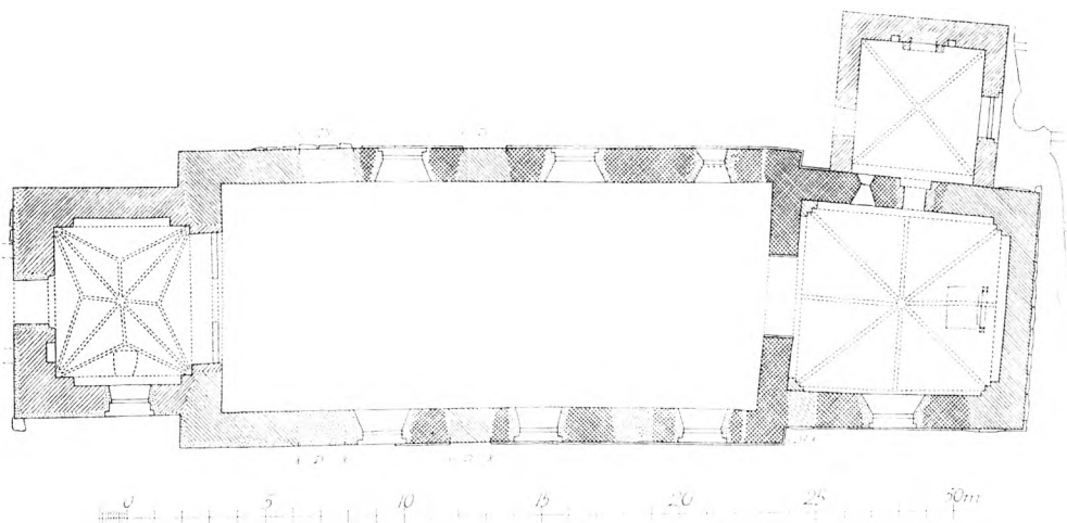
Fig. 2. Øster-Løgum. Plan 1:300. Målt af El. M. 1956.
