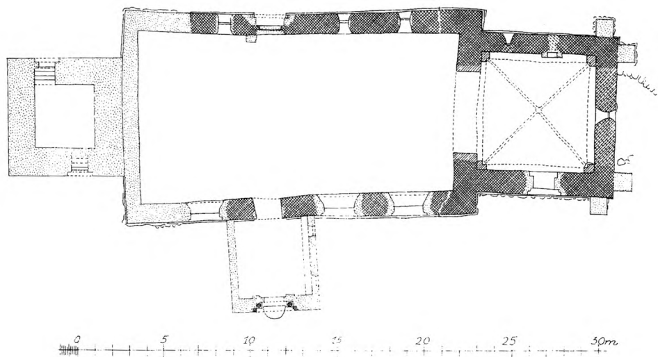
Fig. 2. Bov. Plan 1:300. Målt af H. H. Olrik 1956.
