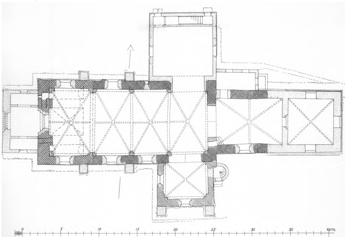
Fig. 3. Nordborg. Plan 1: 300. Målt af H. H. Olrik 1957.
