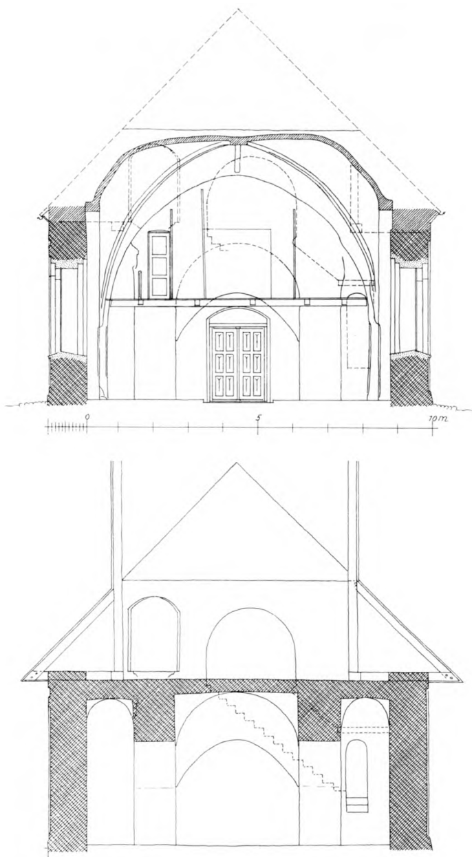
Fig. 2 a—b. Nordborg kirke, a, tværsnit, set mod vest, i den romanske tårnunderdel, der nu indgår som en vestlig, gotisk hvælvet forlængelse af skibet. 1:150. Målt af Palle Friis 1960. b, rekonstruktion (ved El. M.) af det romanske tårns \ddagger hvælv og \ddagger træoverbygning.
