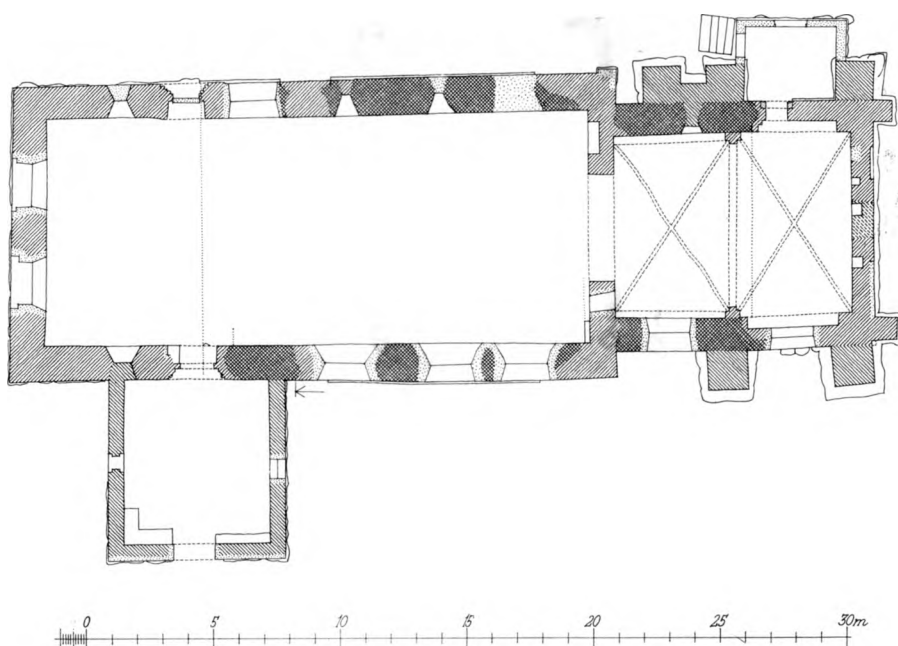
Fig. 2. Hørup. Plan. 1:300. Målt af John Petersen 1957. Tegnet af Holger Schmidt 1961.
