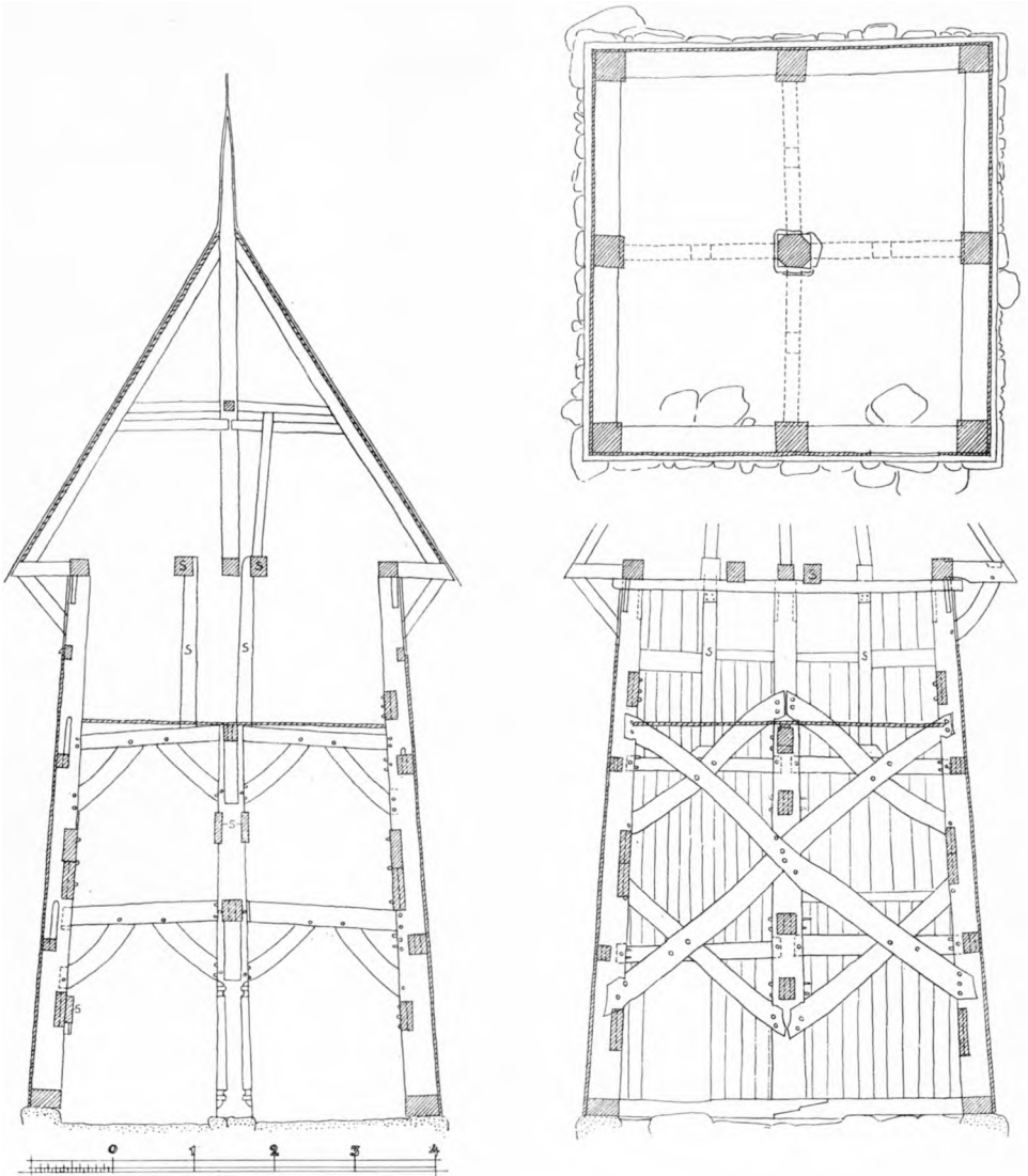
Fig. 3. Tandslet. Klokkehus. Plan, nordvæg og snit langs kongen, set mod nord. 1:100. Målt af El. M. 1959.
