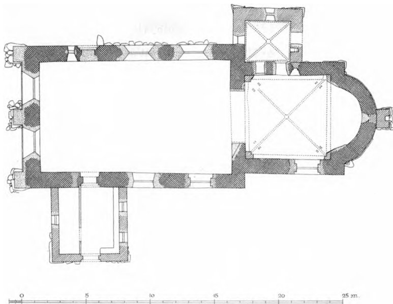
Fig. 2. Tandslet. Plan. 1:300. Målt af C. G. Schultz 1938 (suppleret af El. M. 1960).
