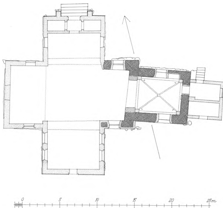
Fig. 2. Asserballe. Plan. 1:300. Målt af John Petersen 1958. Tegnet af Holger Schmidt 1961.
