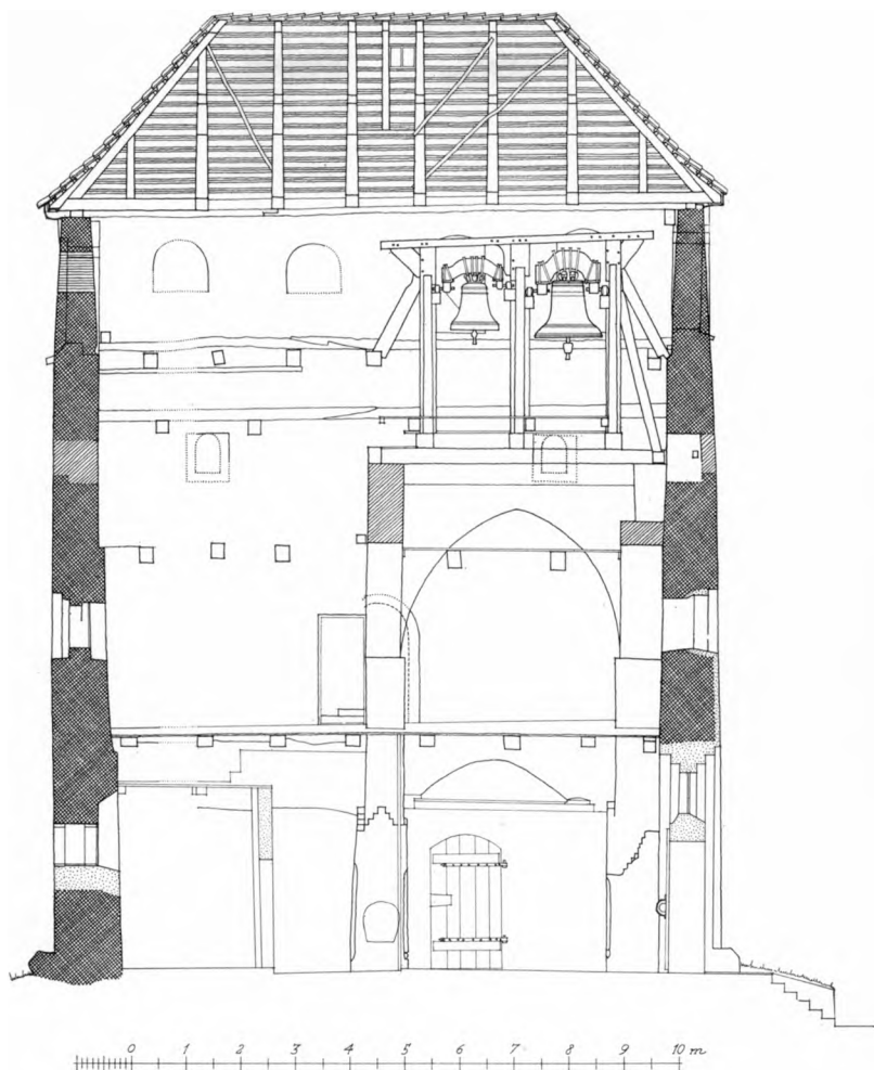
Fig. 5. Ketting. Snit i tårnet, set mod øst. 1:150. Målt af Holger Schmidt 1960.
