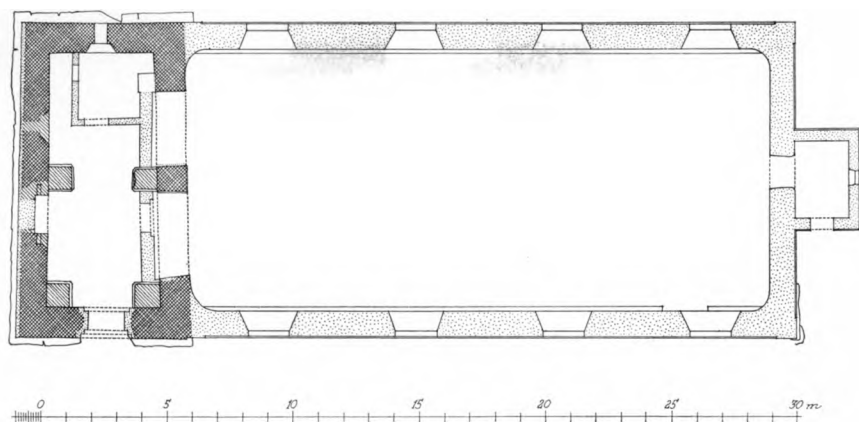
Fig. 2. Ketting. Plan. 1:300. Målt af John Petersen 1958. Tegnet af Holger Schmidt 1961.
