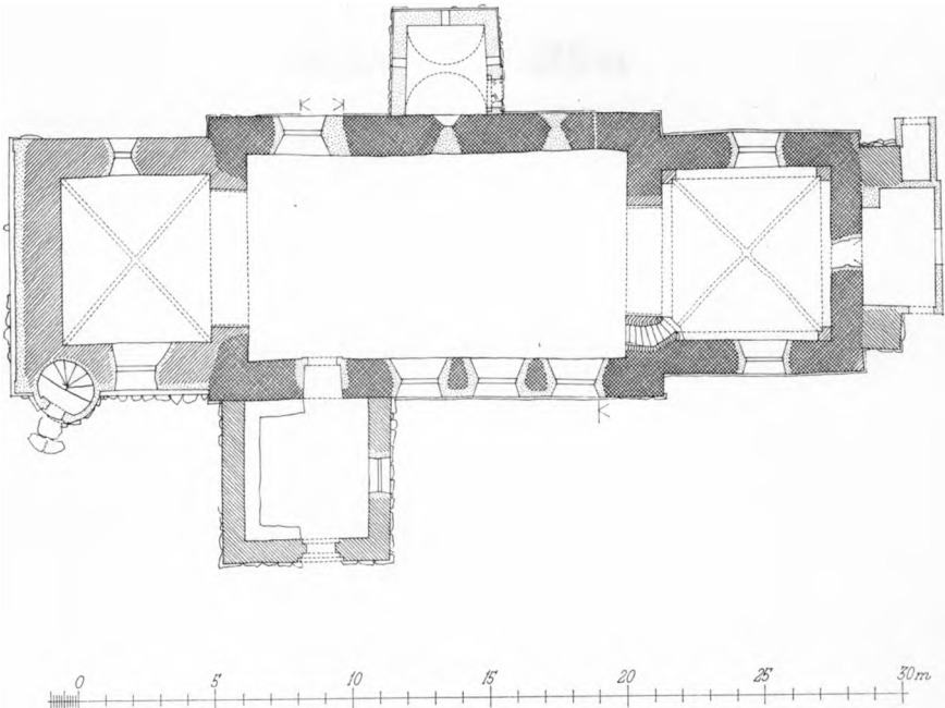
Fig. 2. Oksbøl. Plan. 1:300. Målt af John Petersen 1958.
