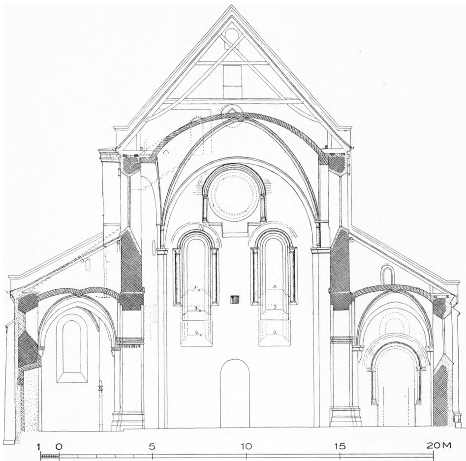
Fig. 7. Sorø. Tværsnit af Midtskibets og Sideskibenes Vestfag (S. 26, 29, 51), set mod Vest; Side skibsportalen delvis rekonstrueret. 1:200. Maalt af Charles Christensen 1933—35.
