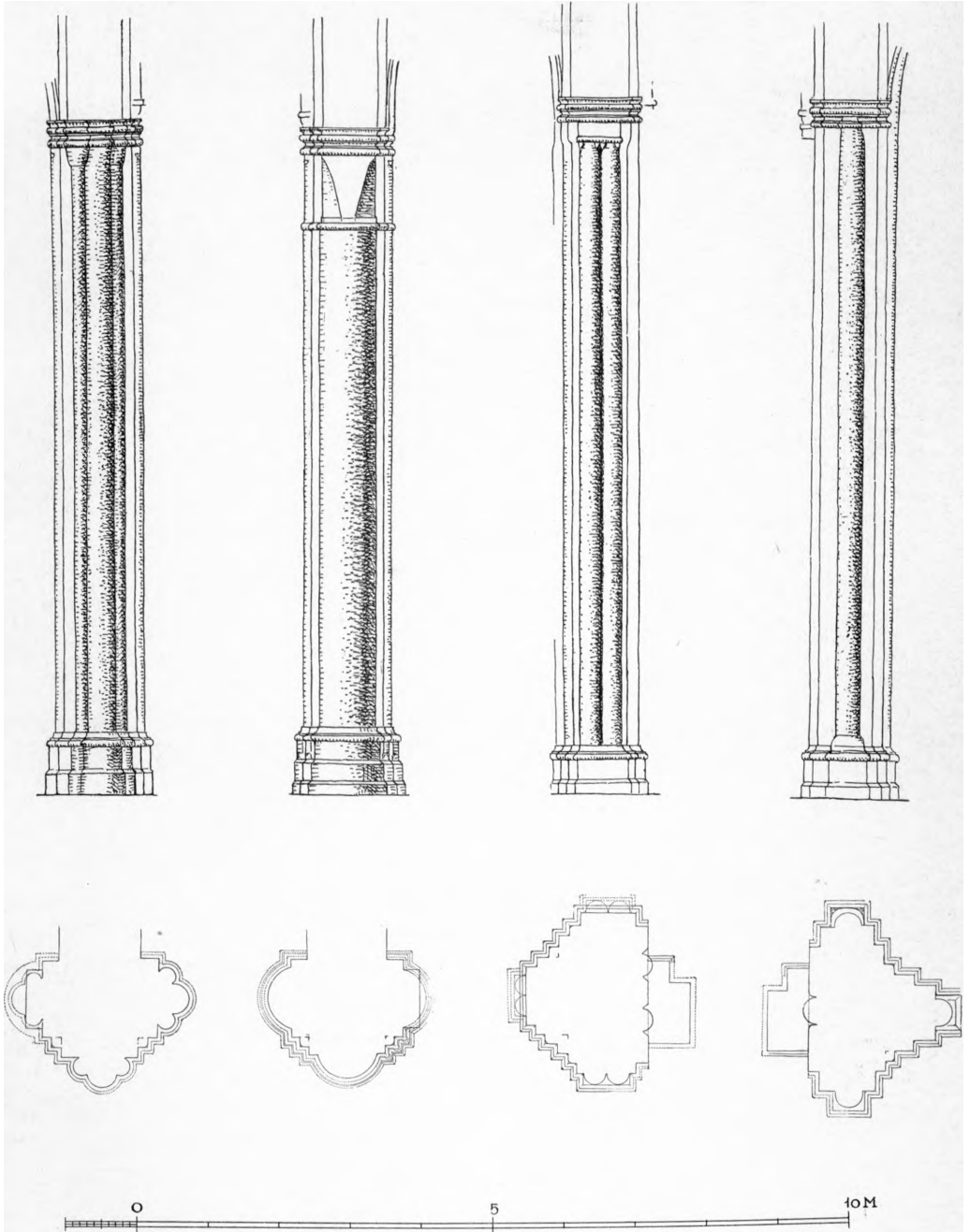
Fig. 13. Sorø. Korsskæringens Piller (S. 31). Fra venstre: den nordøstre og sydøstre, begge set fra Vest; den sydvestre og nordvestre, begge set fra Øst. 1:100. Maalt af Charles Christensen 1933—35.
