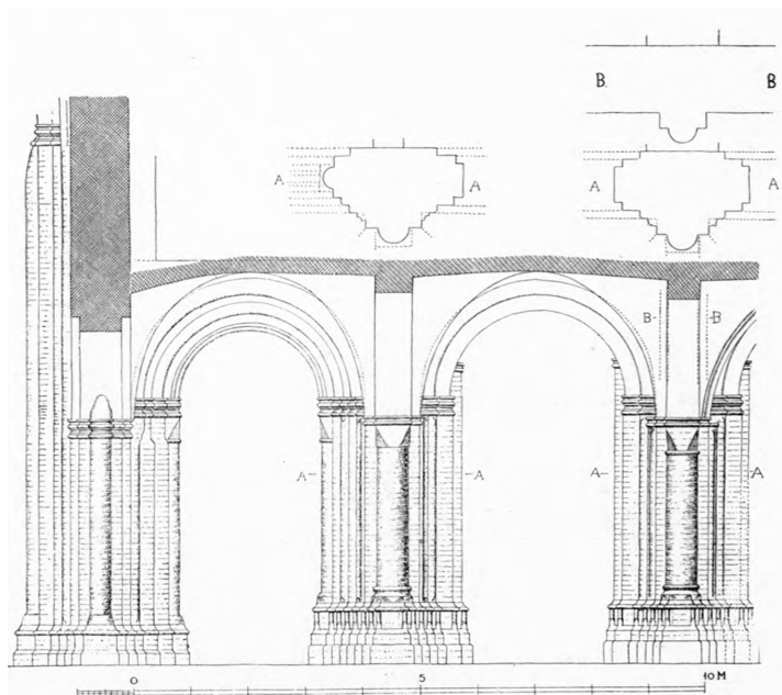
Fig. 10. Sorø. De samme Arkader (S. 34), set fra nordre Sideskib. 1:150. Maalt af Charles Christensen 1933—35.
