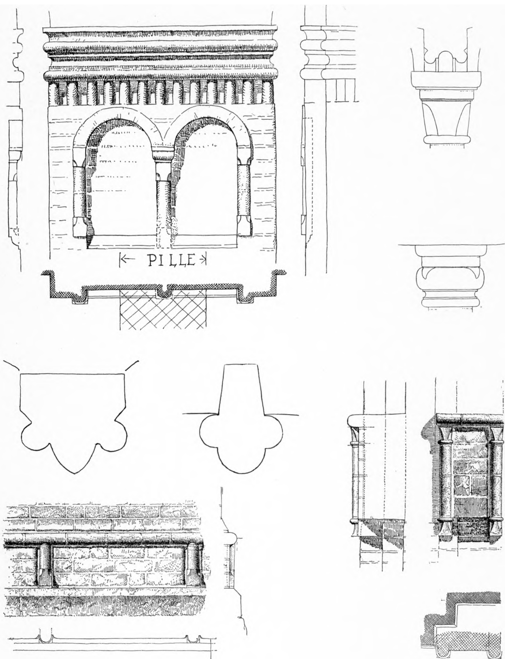
Fig. 12. Sorø. Enkeltheder af Murværk. 1:25. Maalt af Charles Christensen 1933—35.
