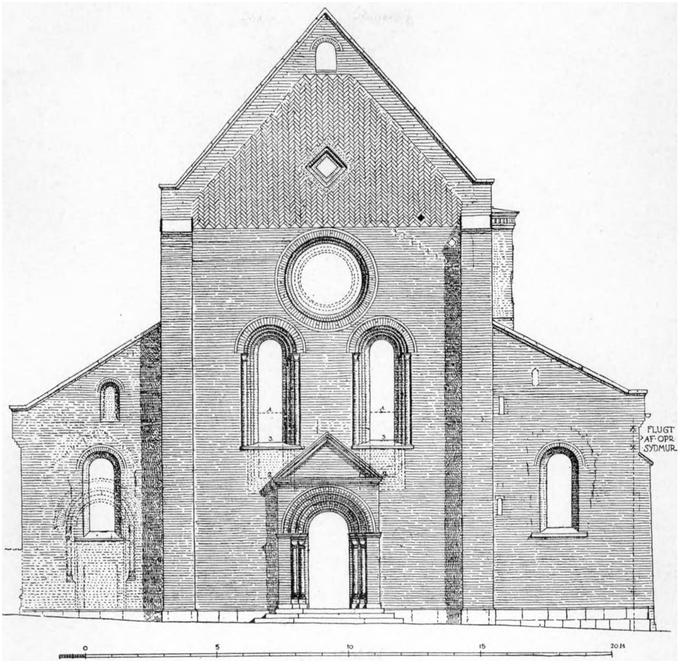
Fig. 8. Sorø. Vestgavl (S. 25, 26); med den rekonstruerede Sideskibsportal indtegnet. 1:200. Maalt af Charles Christensen 1933—35.
