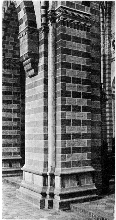
Fig. 17. Sorø. Arkadepille i Søndre Sideskib (S. 35).
