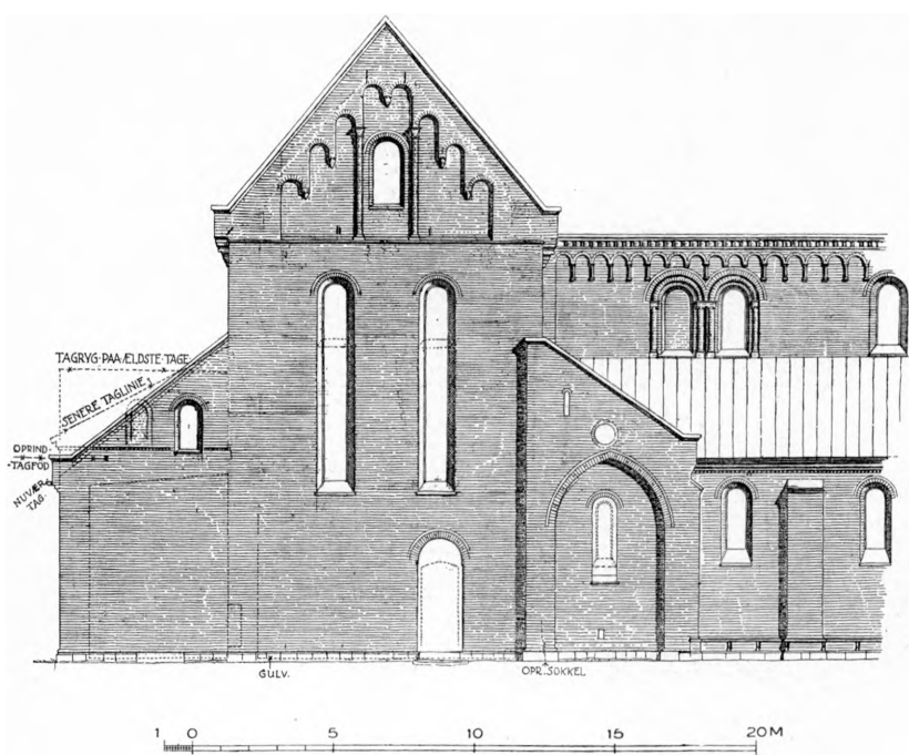
Fig. 5. Sorø. Nordre Korsarm og Østpartiet af Hoved- og Sideskibets Nordmur (S. 28, 44). 1:300. Maalt af Charles Christensen 1933—35.
