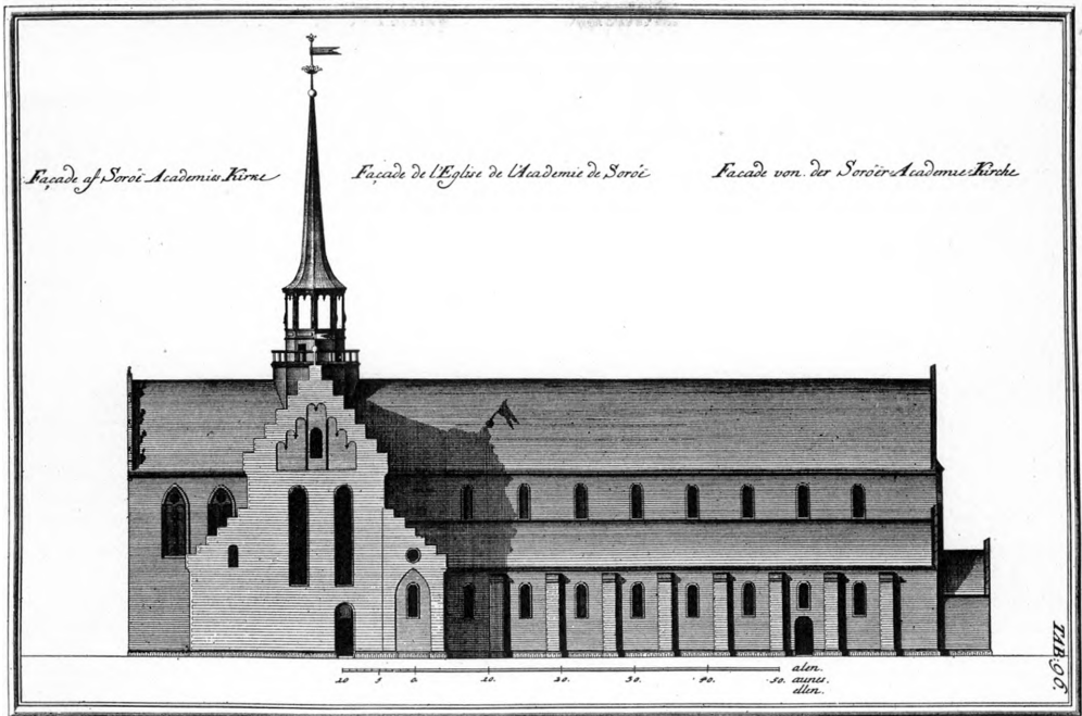
Fig. 25. Sorø. Kirkens Nordfaçade (S. 25, 47, 48). Efter Danske Vitruvius, 1749.
