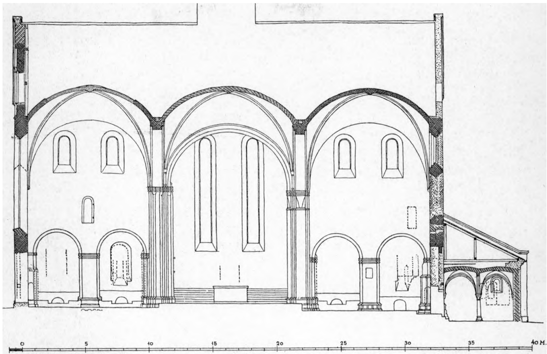
Fig. 6. Sorø. Tværnsnit af Korsskæring og Korsarme (S. 27, 30, 50) set mod Øst. 1:300. Maalt af Charles Christensen 1933—35.
