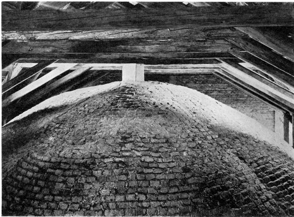
Fig. 19. Sorø. Oversiden af Hvælvet i Søndre Korsarm (S. 39).
