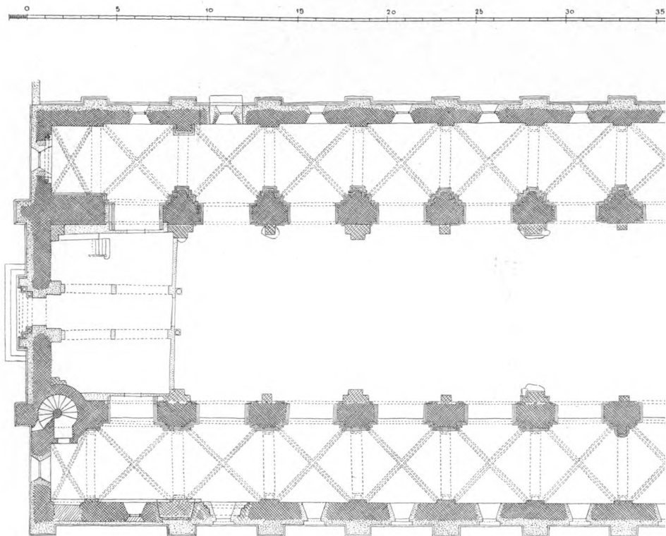
Fig. 4. Soro. Plan. 1:300. Maalt af Charles Christensen 1933—35.
