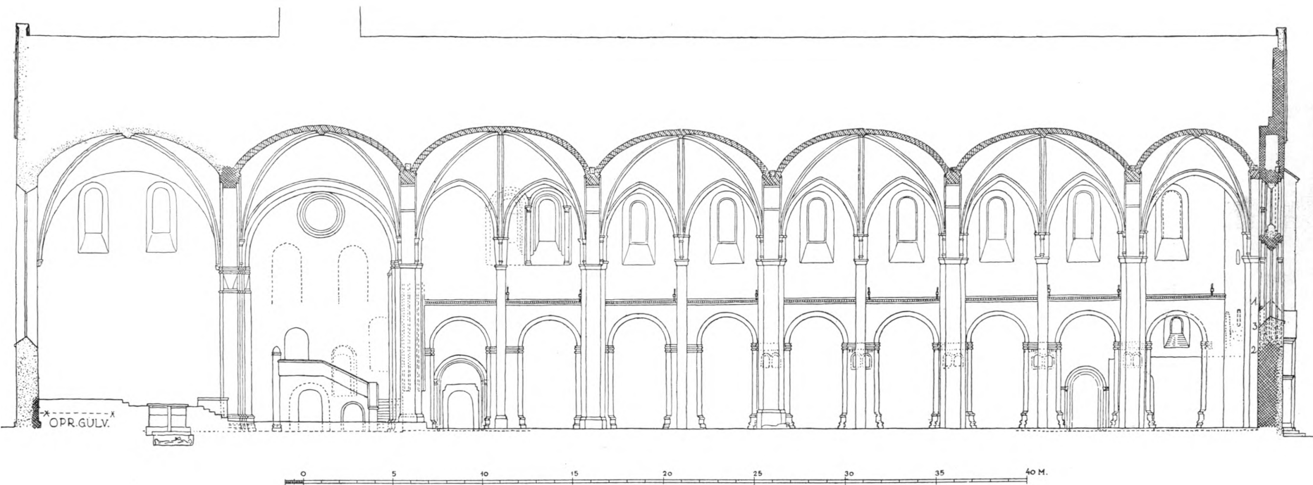
Fig. 11. Sorø. Længdesnit (S.26, 27, 30, 50, 79), set mod Syd, med de delvis rekonstruerede Portaler indtegnet. 1: 300. Maalt af Charles Christensen 1933—35.
