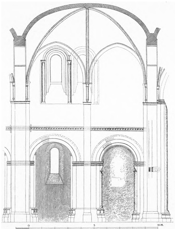
Fig. 9. Sorø. Skibets to østligste Arkader (S. 28), set mod nordre Sideskib. 1:150. Maalt af Charles Christensen 1933—35.
