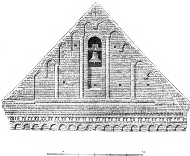
Fig. 11. Ringsted. Nordre Korsarms Gavl. 1:150. Efter Clemmensen.
