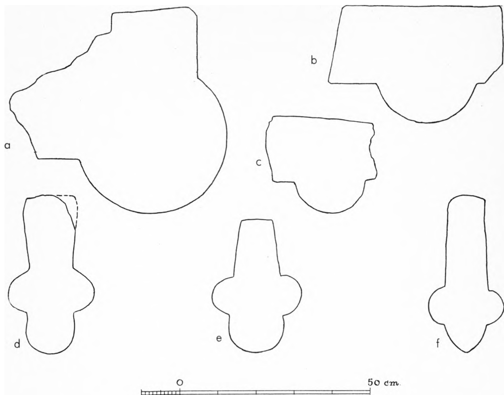
Fig. 17. Ringsted. Formsten. 1:10. a—d: af Fraadsten (S. 112), e—f: af Tegl (S. 133). Maalt af C. G. Schultz 1935.
