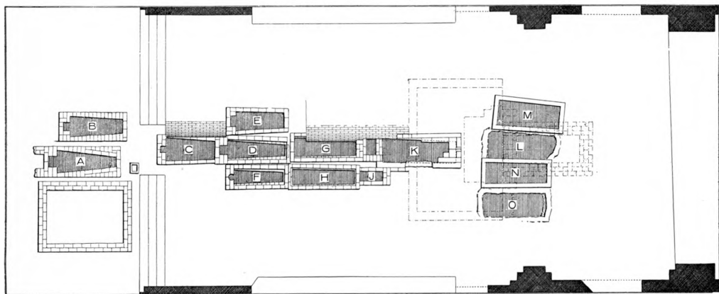
Fig. 45. Ringsted. Plan over Kongegravene, ca. 1:175. Øst til højre.
