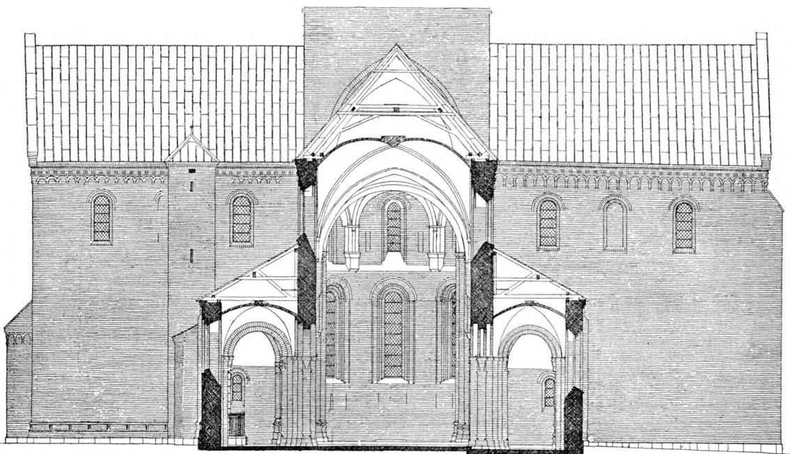
Fig. 13. Ringsted. Tværsnit af Skibet, set mod Øst. 1:300. Efter Clemmensen.
