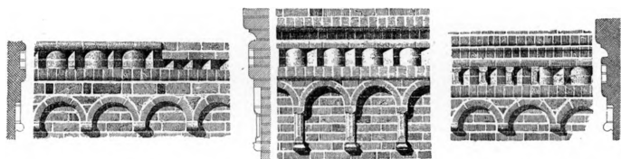
Fig. 4. Ringsted. Gesims. 1:75. I Midten: Korets Gesims. Tilvenstre: Gesims paa Skibets Syd-side ved Skellet mellem to Byggeperioder (S. 122, 129). Tilhøjre: Gesims paa Nordre Korsarms Gavl. Efter Clemmensen.
