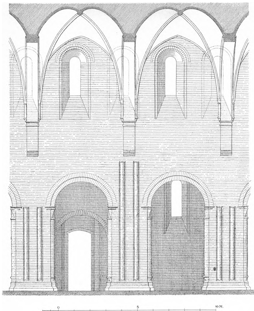
Fig. 15. Ringsted. Fjerde og femte Fag af Midtskibets Nordside (S. 130 ff.). 1:150. Efter Clemmensen.
