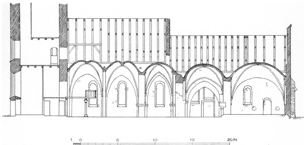
Fig. 4. Slagelse. S. Peder. Længdesnit, set mod Nord. 1:300. Før Istandsættelsen. Maalt af Herholdt.
