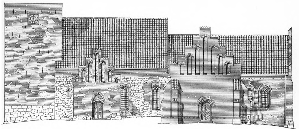
Fig. 3. Slagelse. S. Peder. Syd façade. 1: 300. Før Istandsættelsen. Maalt af Herholdt.
