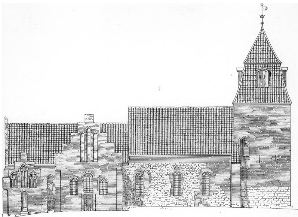
Fig. 5. Slagelse. S. Peder. Nordfaçade. 1:300. Før Istandsættelsen. Maalt af Herholdt.
