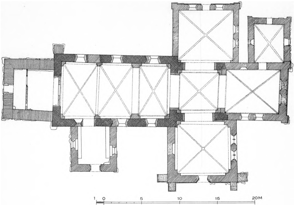
Fig. 2. Slagelse. S. Peder. Plan. 1:300. Maalt af Arne Nystrom 1930.
