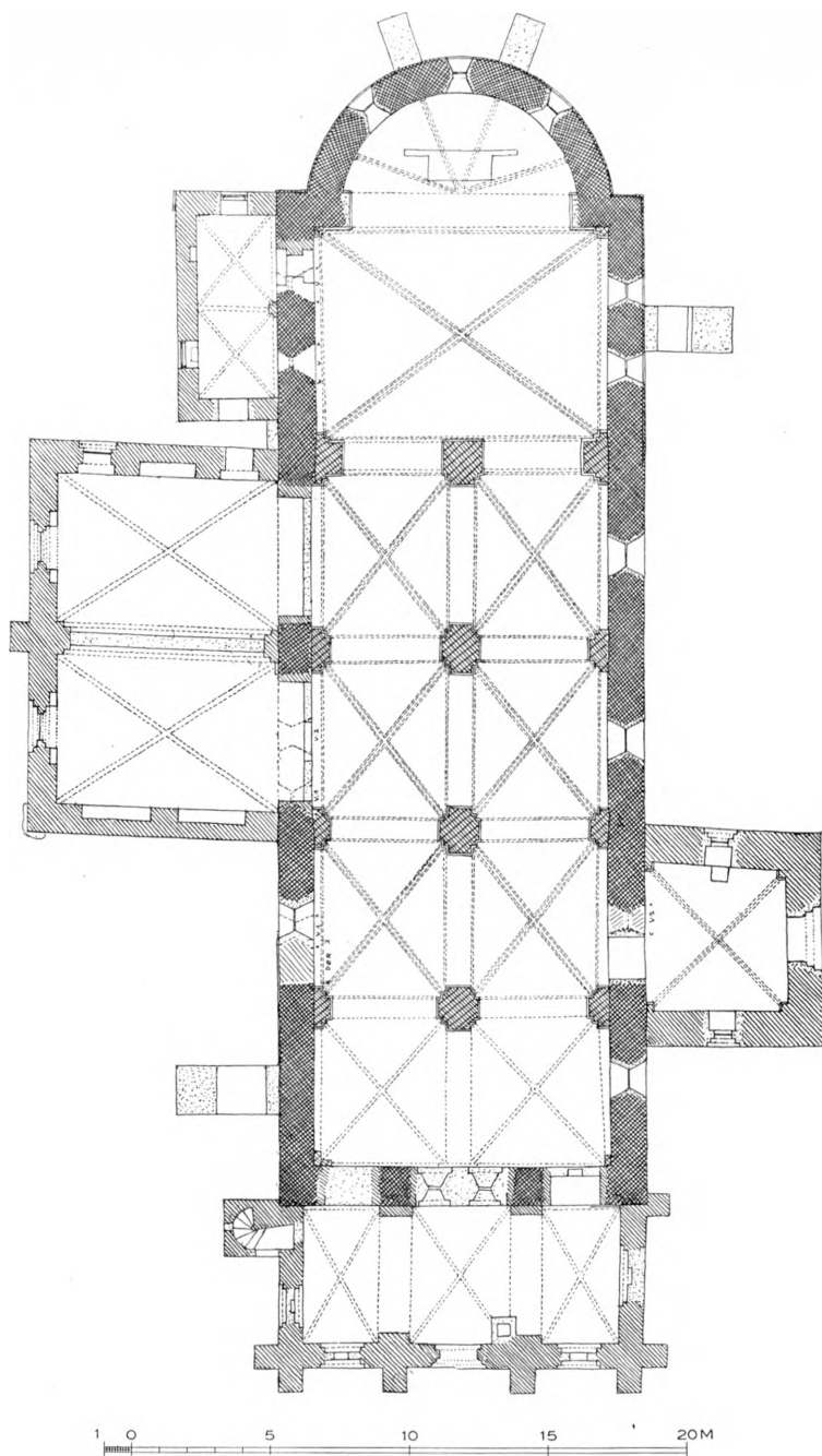
Fig. 4. Skelskør. Plan. 1:300. Ost opad. Maalt af Charles Christensen 1929.
