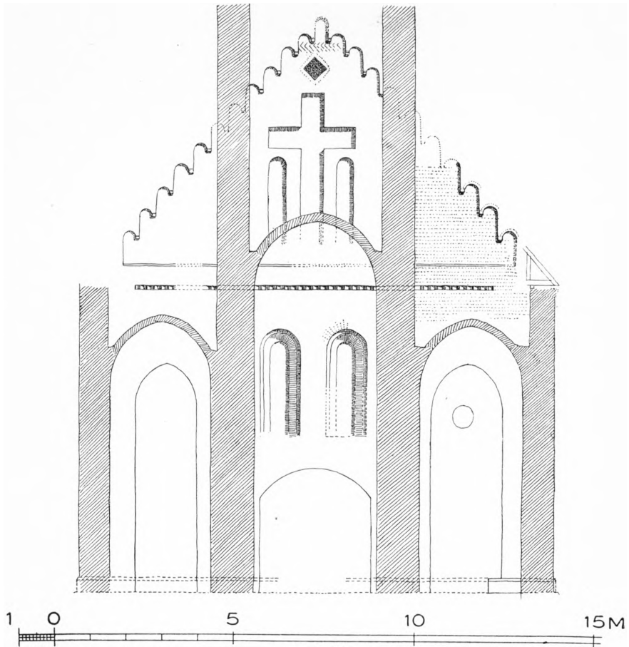
Fig. 5. Skelskør. Skibets Vestgavl og Snit gennem Taarnet. 1:150. Maalt af Charles Christensen 1929.
