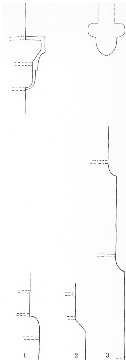
Fig. 7. Skelskør. Profiler. 1:10. Foroven t. v.: Kragbaand, fra en Midt-skibspille, med moderne Puds-Profil (S. 251); t. h.: Ribbesten (S. 247). Forneden: Sokkelprofiler (S. 242). 1. Skibets Nordmur, 2. Vestgavlen, 3. Koret.
