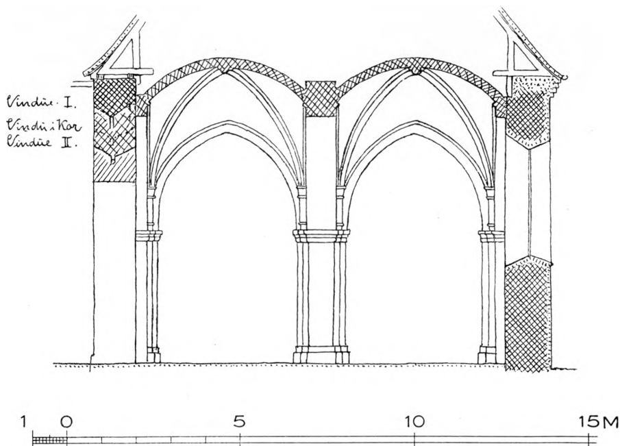
Fig. 6. Skelskor. Tværsnit gennem Skibet, set mod Ost. 1:150. Maalt af Charles Christensen 1929.
