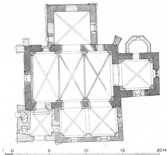
Fig. 3. Pedersborg. Plan. 1:300. Maalt af Charles Christensen 1930.
