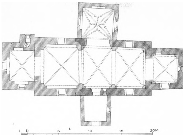
Fig. 2. Lyng. Plan. 1:300. Maalt af C. G. Schultz 1931.
