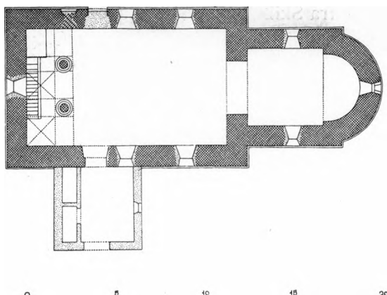
Fig. 2. Kirke-Fjenneslev. Plan. 1:300. Maalt af C. G. Schultz 1931.
