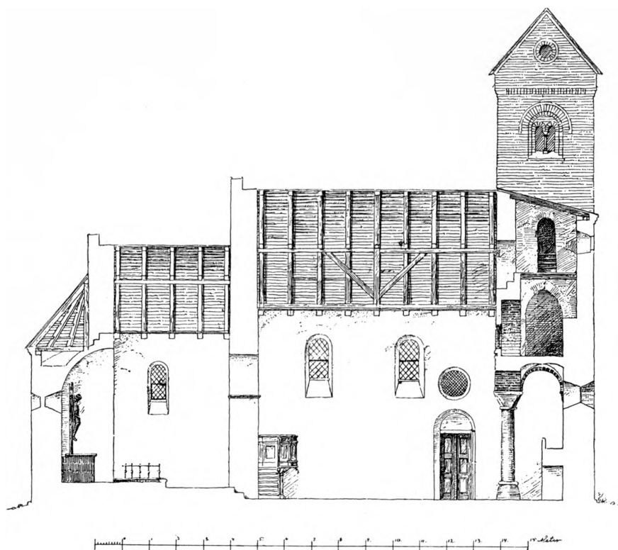
Fig. 4. Kirke-Fjenneslev. Længdesnit, 1:200, set mod Syd. Maalt af H. B. Storck 1893.
