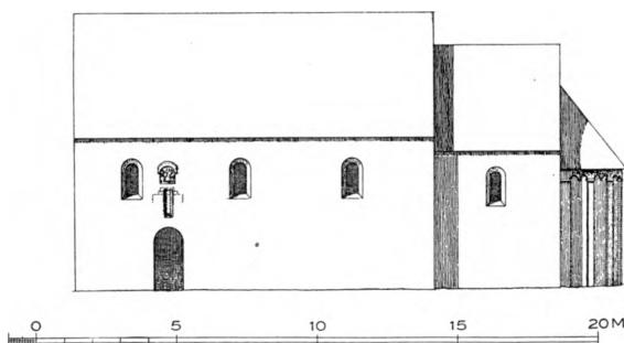
Fig. 3. Slaglille. Syd façade af den romanske Kirke. 1:300. Rekonstruktionsopmaaling af C. G. Schultz 1931.
