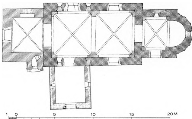
Fig. 2. Slaglille. Plan. 1:300. Maalt af C. G. Schultz 1931.
