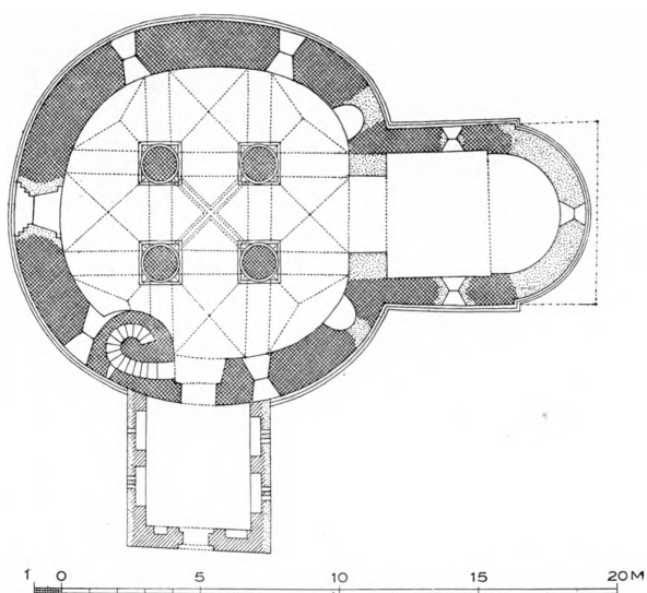
Fig. 2. Bjernede. Plan. 1:300. Maalt af C. G. Schultz 1931.
