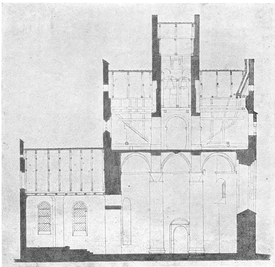
Fig. 4. Bjernede. Længdesnit, før Restaureringen, set mod Syd. 1:200. Maalt af H. B. Storck 1887.
