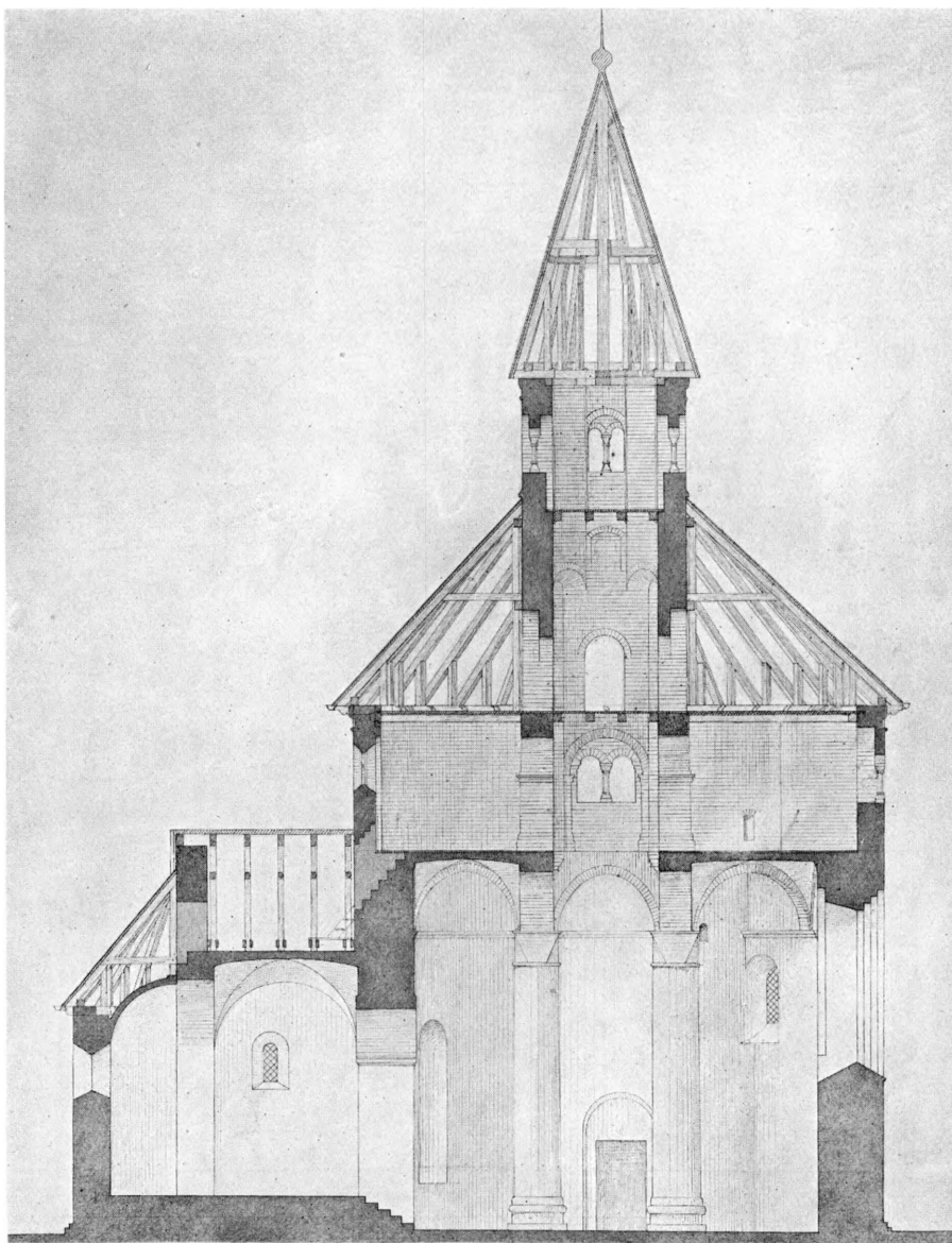
00. H. B. Storcks Arbejdstegning 1887 for Restaureringen. Midthvælvingen var paatænkt fjernet, men blev bibeholdt, da det under Restaur
