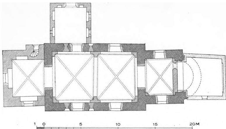
Fig. 2. Gyrstinge. Plan. 1:300. Maalt af C. G. Schultz 1931.
