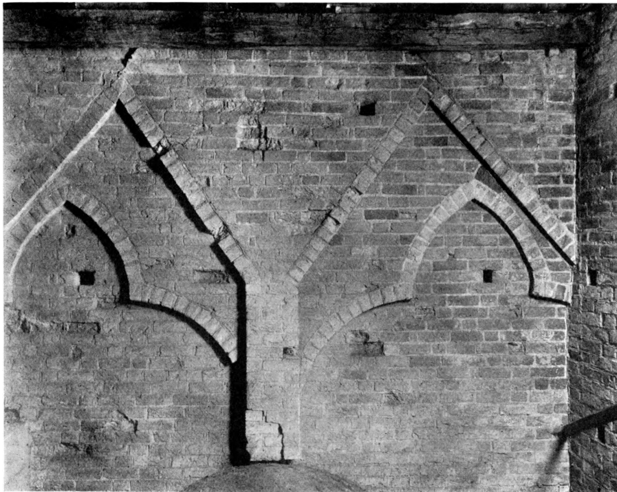
Fig. 4. Benløse. Skibets Vestgavl. (S. 414).
