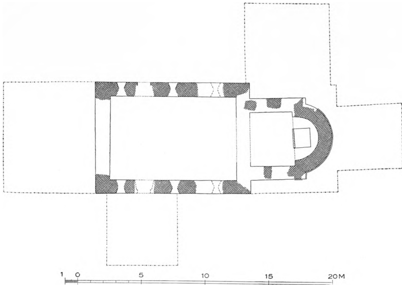
Fig. 3. Bringstrup. Plan. 1:300. Maalt af C. G. Schultz 1930. De i Mur og Fundament bevarede romanske Dele.
