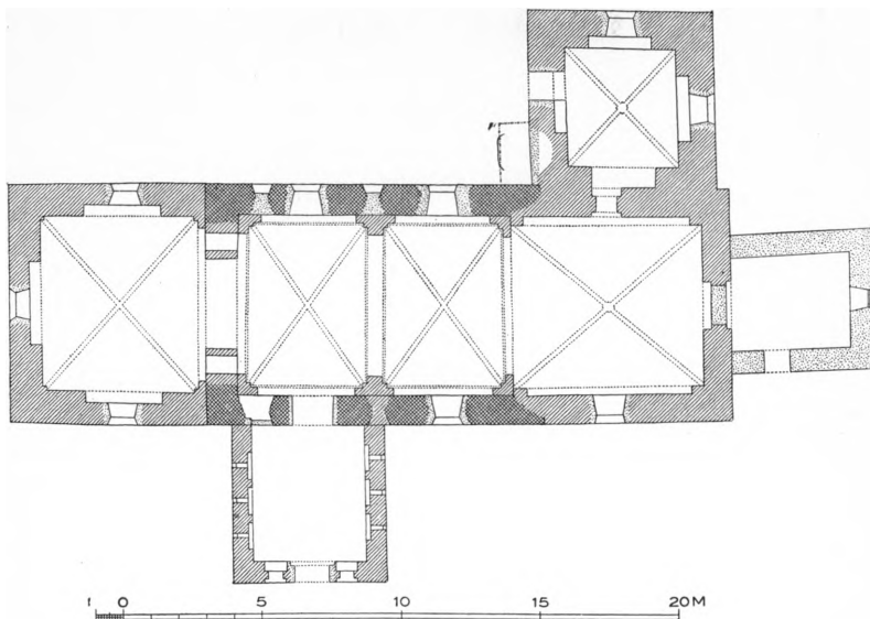
Fig. 2. Bringstrup. Plan. 1:300. Maalt af C. G. Schultz 1930.
