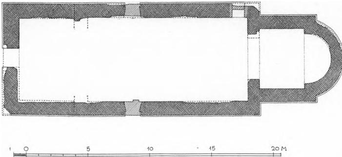
Knud Lavards Kapel. Plan. 1:300. Maalt af J. B. Løffler 1884 (C. G. Schultz 1930).
