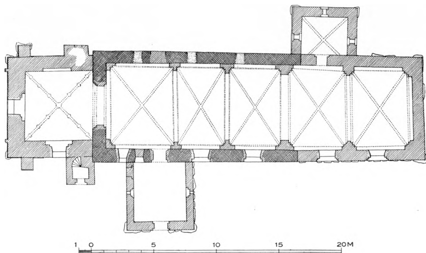
Fig. 2. Haraldsted. Plan. 1:300. Maalt af Aage Roussell 1929.
