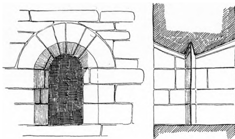
Fig. 3. Haraldsted. Romansk Vindue i Skibets Sydmur. Yderside og Snit. 1:50. Maalt af K. V. Barfoed 1913. (S. 444).
