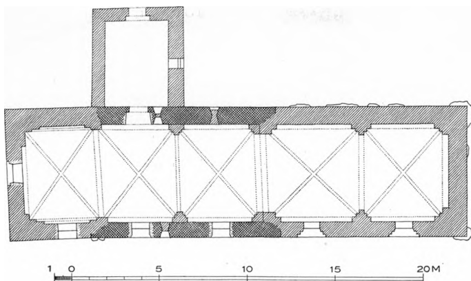
Fig. 2. Allindemagle. Plan, 1:300. Maalt af K. V. Barfoed 1913. (C. G. Schultz 1930).
