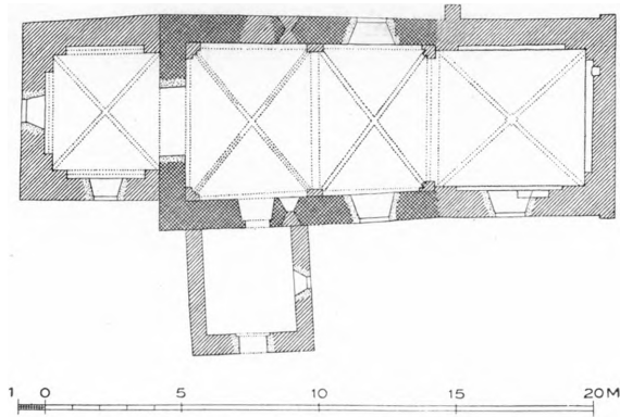
Fig. 2. Jydstrup. Plan. 1:300. Maalt af Mogens Clemmensen 1917.
