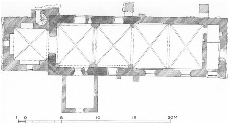
Fig. 2. Vigersted. Plan. 1 : 300. Maalt af Mogens Clemmensen 1917.
