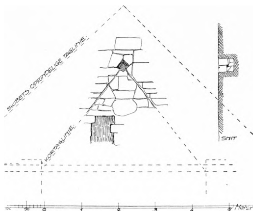
Fig. 3. Kværkeby. Skibets Østgavl, set mod Vest (S. 498). 1:100. Maalt af IC. V. Barfoed 1913.
