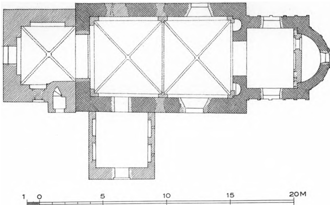
Fig. 2. Kværkeby. Plan. 1:300. Maalt af K. V. Barfoed 1913 (C. G. Schultz 1931).
