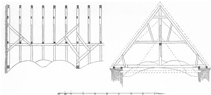
Fig. 4. Kværkeby. Langsnit og Tværsnit af Skibets Tagværk (S. 499). 1 : 150. Maalt af K. V. Barfoed 1913.
