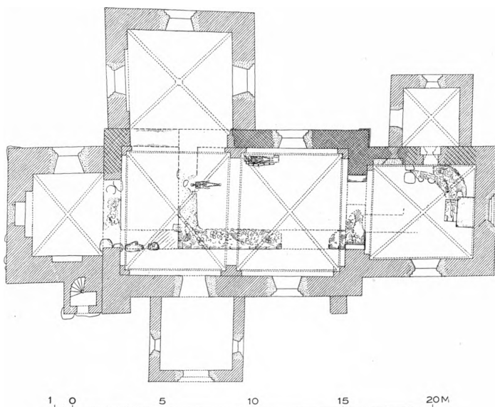
Fig. 2. Haslev før Ombygningen 1914—16. Plan. 1 : 300. Tegnet af C. G. Schultz 1936 paa Grundlag af Th. Havnings, M. Clemmensens og C. A. Jensens Opmaalinger.
