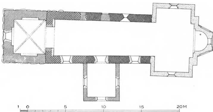
Fig. 2. Freerslev. Plan. 1: 300. Maalt af C. G. Schultz 1930.
