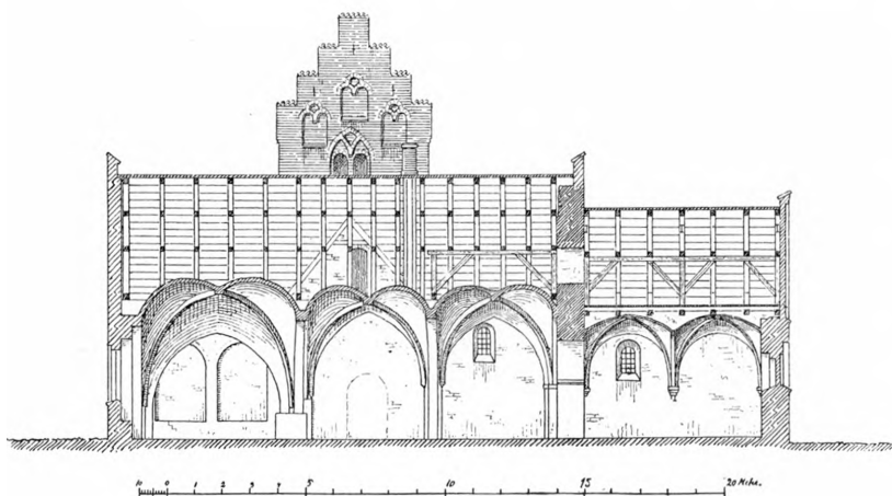
Fig. 5. Sønderup. Længdesnit, set mod Nord. 1 : 300. Maalt af F. C. C. Hansen 1892.
