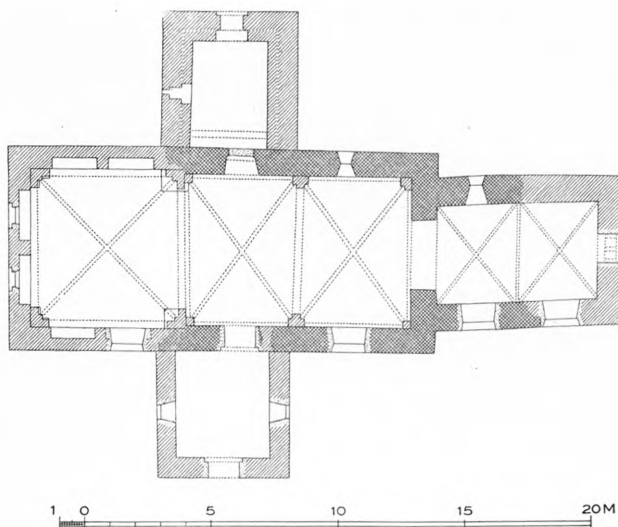
Fig. 2. Sönderup. Plan. 1 : 300. Maalt af F. C. C. Hansen 1892 (C. G. Schultz 1931).
