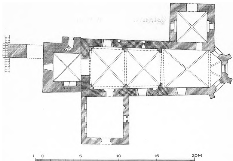
Fig. 2. Slots-Bjærgby. Plan. 1 : 300. Maalt af K. V. Barfoed 1915 (Aage Roussell 1932).
