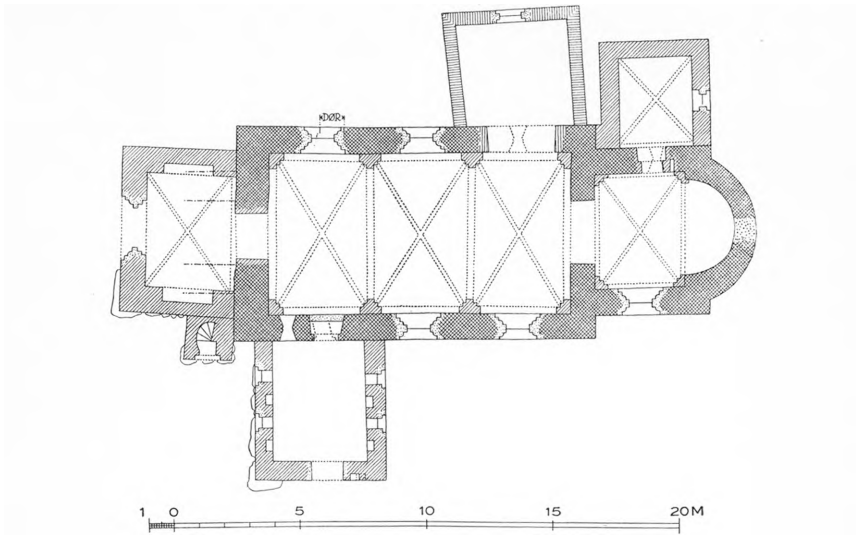
Fig. 2. Sludstrup. Plan. 1 : 300. Maalt af K. V. Barfoed 1915 (C. G. Schultz 1931).
