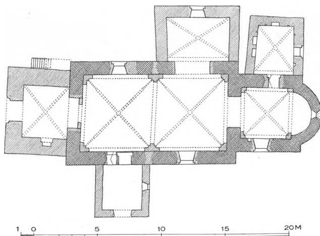
Fig. 2. Lundforlund. Plan. 1 : 300. Maalt af K. V. Barfoed 1915 (Aage Roussell 1932).
