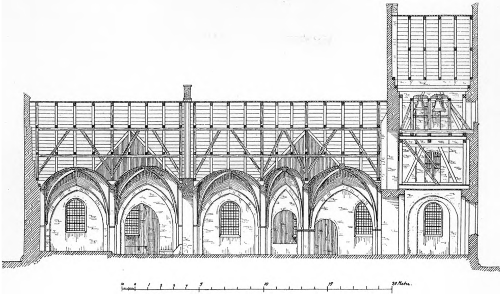
Fig. 3. Kirke-Stillinge. Længdesnit, set fra Nord. 1 : 300. Maalt af F. C. C. Hansen 1892.
