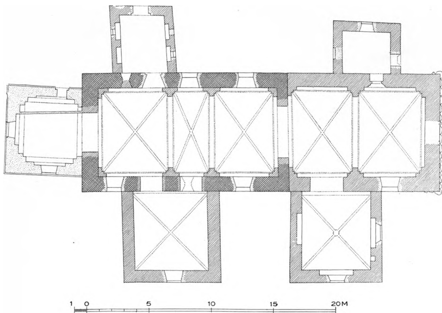
Fig. 2. Kirke-Stillinge. Plan. 1 : 300. Maalt af F. C. C. Hansen 1892 (C. G. Schultz 1932).
