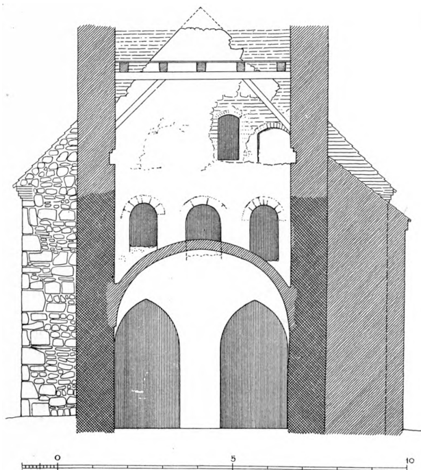
Fig. 7. Eggeslevmagle. Skibets gamle Vestgavl (S. 778) og Snit gennem Taarnet, set mod Øst. 1:150. Maalt af C. G. Schultz 1938.
