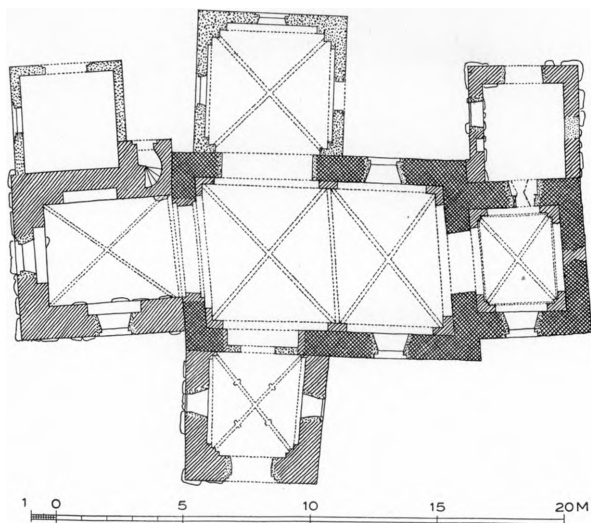
Fig. 2. Flakkebjerg. Plan. 1:300. Maalt af Arne Nystrom 1928.
