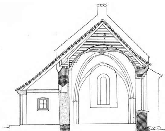
Fig. 3. Skørpinge. Tværnsnit gennem Koret i dets nuværende Tilstand, set mod Øst. 1:150. Maalt af C. G. Schultz 1938.
