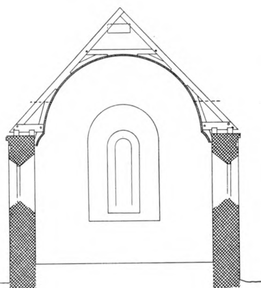
Fig. 4. Skørpinge. Tværnsnit gennem det romanske Ivor, set mod Øst. 1:150. Rekonstruktion af C. G. Schultz 1938.
