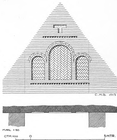
Fig. 6. Skørpinge. Skibets romanske Vestgavl. 1:150. Maalt af C. M. Smidt 1913 (S. 810).
