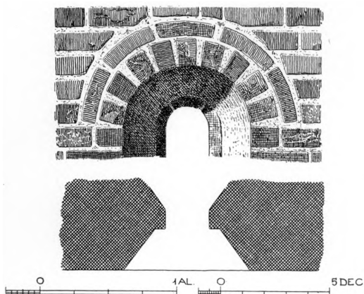
Fig. 5. Skørpinge. Romansk Vindue i Skibets Sydmur. 2:5. Maalt af C. M. Smidt 1913 (S. 809).
