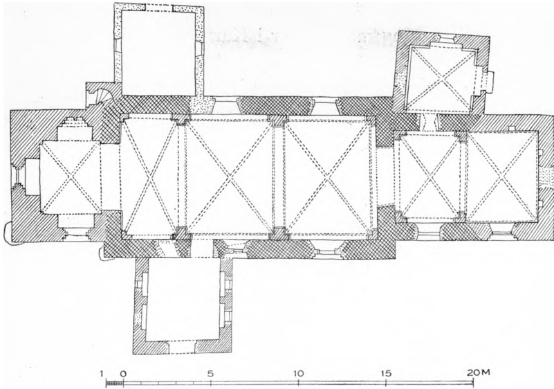
Fig. 2. Gimlinge. Plan. 1:300. Maalt af Charles Christensen 1932.
