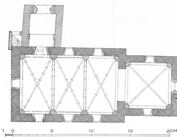
Fig. 2. Haarslev. Plan. 1:300. Maalt af Arne Nystrom 1928.
