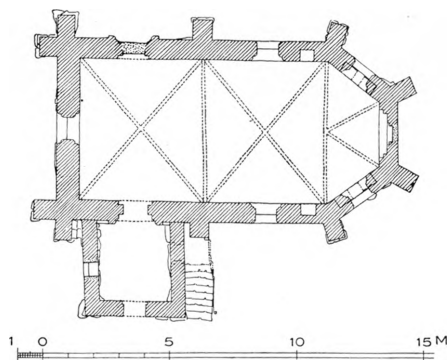
Fig. 2. Ting-Jellinge. Plan. 1 :300. Maalt af Arne Nystrom 1928.
