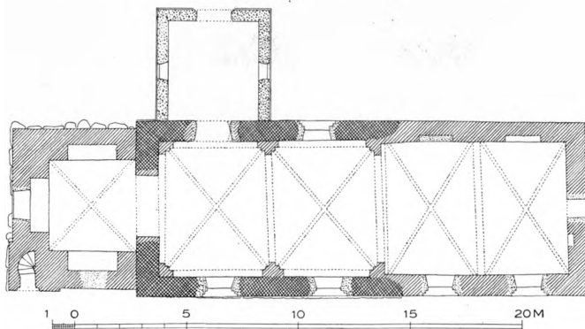
Fig. 2. Sønder Bjærg. Plan. 1:300. Maalt af Arne Nystrom 1928.
