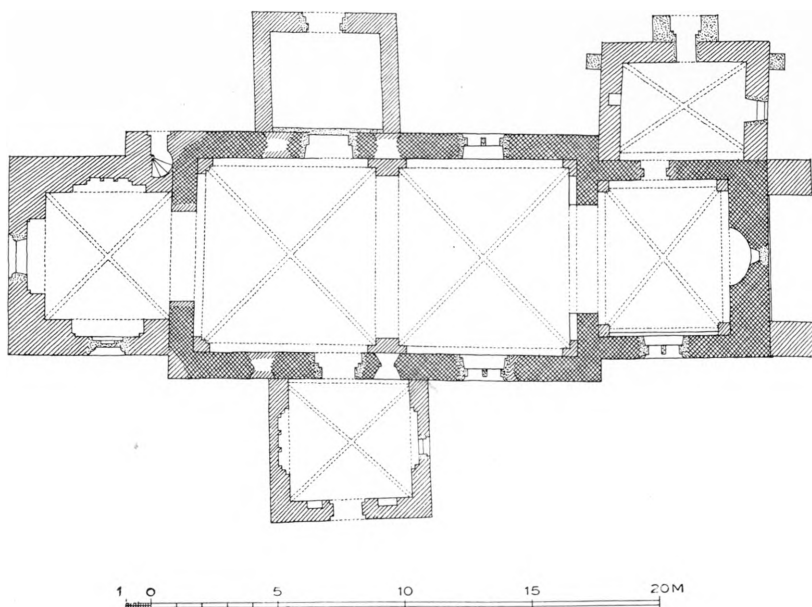
Fig. 2. Tjæreby. Plan. 1:300. Maalt af Arne Nystrom 1931.
