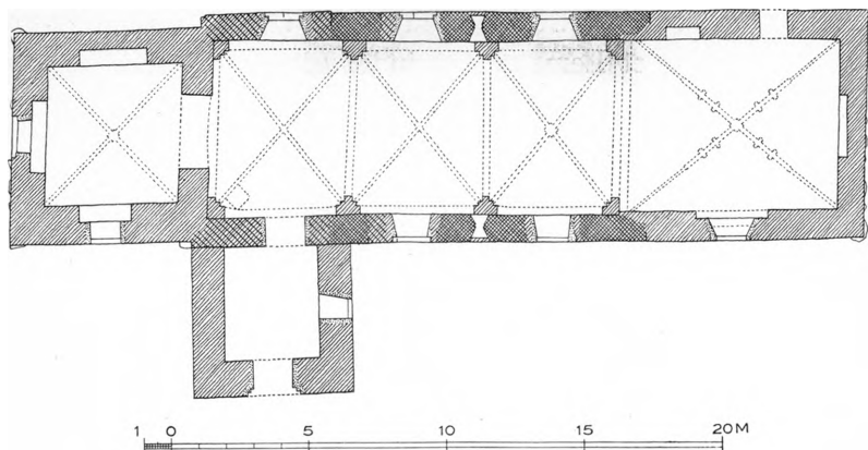
Fig. 2. Krummerup. Plan. 1:300. Maalt af Aage Roussell 1931.
