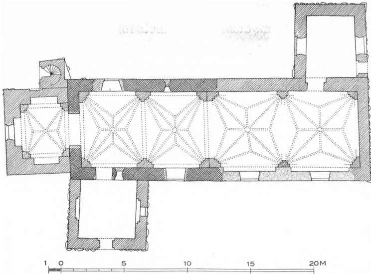
Fig. 2. Hyllinge. Plan. 1 : 300. Maalt af Aage Roussell 1931.
