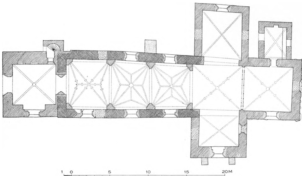
Fig. 2. Fyrendal. Plan. 1 : 300. Maalt af Aage Roussell 1931.
