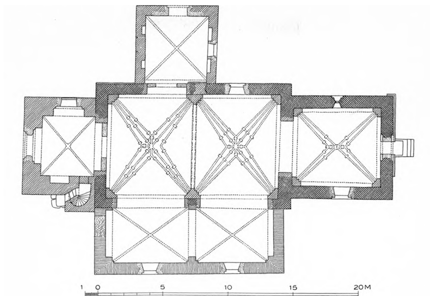
Fig. 2. Karrebæk. Plan. 1 : 300. Maalt af Kristian Rud 1930 (C. G. Schultz 1938).
