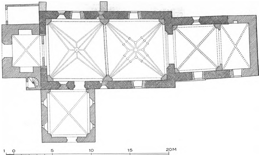
Fig. 2. Fodby. Plan. 1 : 300. Maalt af Kristian Rud (Aage Roussell 1932).
