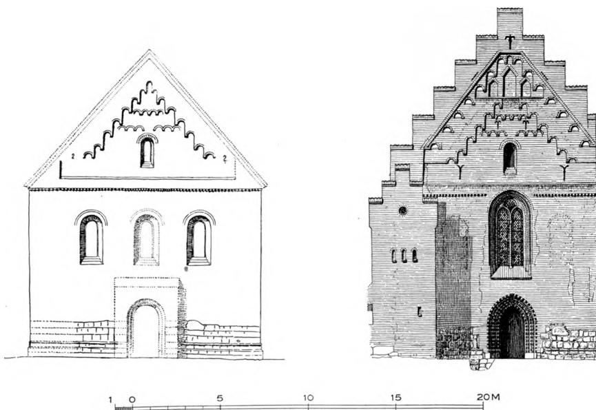
Fig. 6. Herlufsholm. Vestgavl. 1:300. Nuværende Tilstand til højre; Rekonstruktion til venstre. Maalt af Charles Christensen 1929—30 (S. 1118, 1120). Efter V. Lorentzen.
