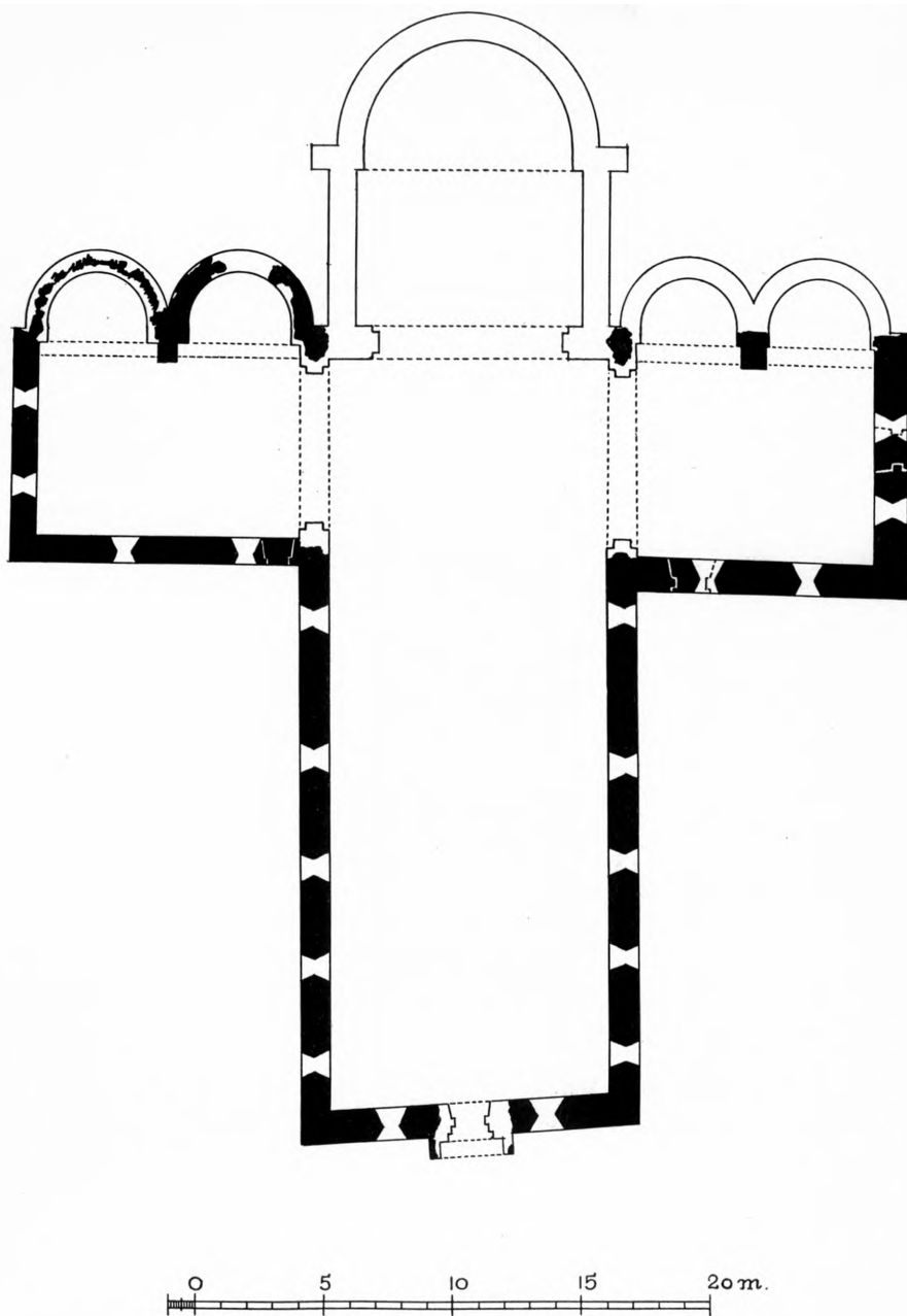
Fig. 3. Herlufsholm. Rekonstruktionsplan af den oprindelige Kirke. 1:300. (C. G. Schultz 1939). Øst opad (S. 1116).
