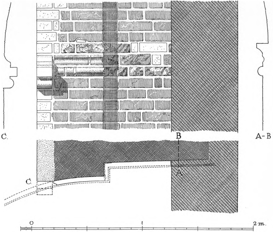
Fig. 8. Herlufsholm. A—B forhugget Kragbaand mod Syd i søndre Korsarms nordre Apsisbue; C et Pynteled fra Herholdts Istandsættelse. Murværket fra denne Restaurering 1861—63 staar lyst. 1 : 20. Maalt af C. G. Schultz 1939 (S. 1119 f.).
