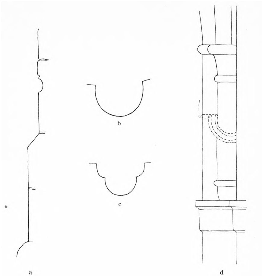
Fig. 15. Herlufsholm, a—c. Profiler. 1 : 10. a. Granit-Sokkel under Vestgavlen, b. Ribber i Skibets to Vestfag, c. Ribber i Kirkens øvrige Hvælvinger. d. Hvælvings-Dværgsøjle. 1 : 20. Maalt af Charles Christensen 1929—30 (S. 1117, 1122).
