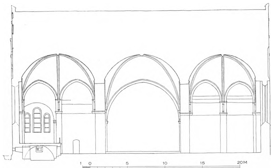
Fig. 12. Herlufsholm. Snit af Korsarme og Kor, set mod Øst. 1 : 300. Maalt af Charles Christensen 1929—30 (S. 1122).
