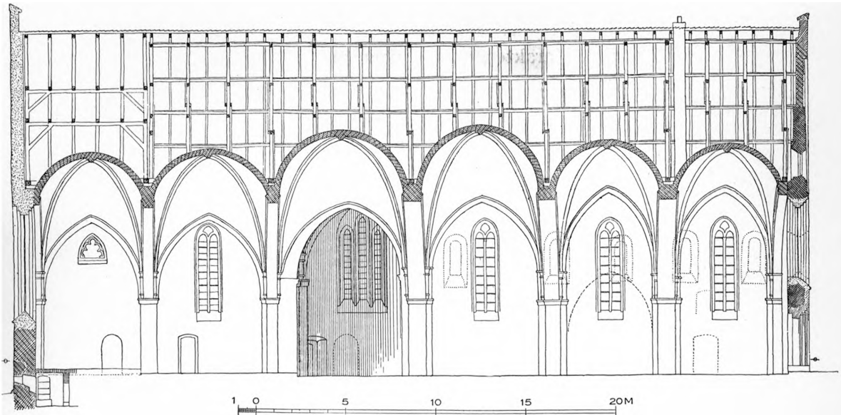
Fig. 14. Herlufsholm. Længdesnit af Skib og Kor, set mod Syd. 1 : 300. Maalt af Charles Christensen 1929—30 (S. 1122 ff.).
