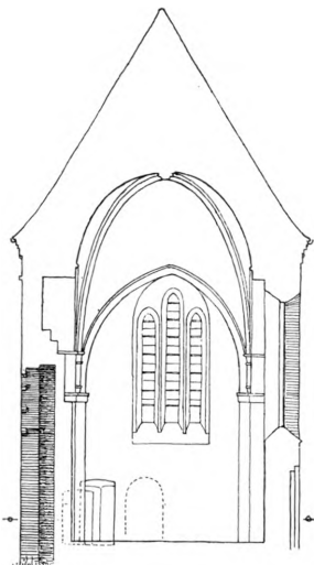
Fig. 10. Herlufsholm. Tværnsnit af søndre Kors- arm, set mod Syd. 1 : 300. Maalt af Charles Christen- sen 1929—30 (S. 1120, 1125).
