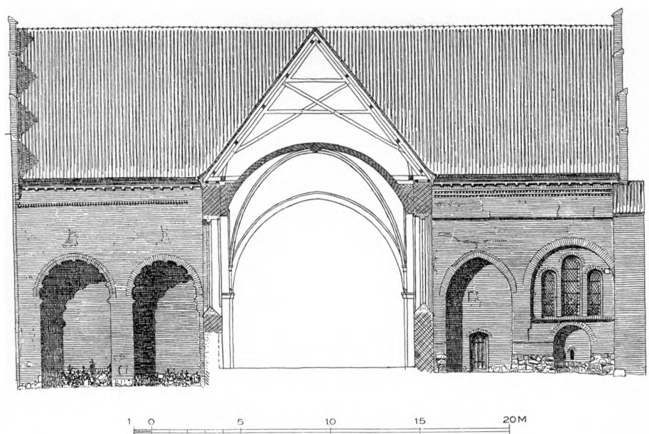
Fig. 11. Herlufsholm. Korsarmenes Østside og Snit af Kor; set mod Vest. 1 : 300. Maalt af Charles Christensen 1929—30 (S. 1120, 1128).
