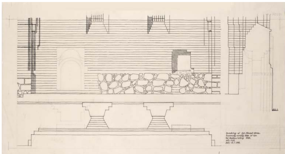
Fig. 26. Opstalt af den nederste del af korets nordvæg. 1:100. Kampestensmurværket forinden er fra den ældre \dagger kirke. Opmåling ved A. Jensen 1949. Danmarks Kunstmuseer. – Drawing of the lower part of the chancel's north side (interior), 1949. The boulders are from earlier \dagger church.
