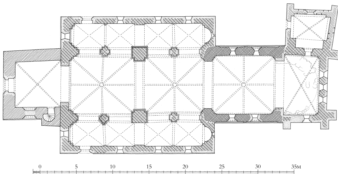
Fig. 29. Grundplan. 1:300. Tegnet af Merete Rude 2011 efter opmåling af Magdahl Nielsen 1898, korrigeret af Marianne Goral Krogh Johansen 2011. – Grundplan.
