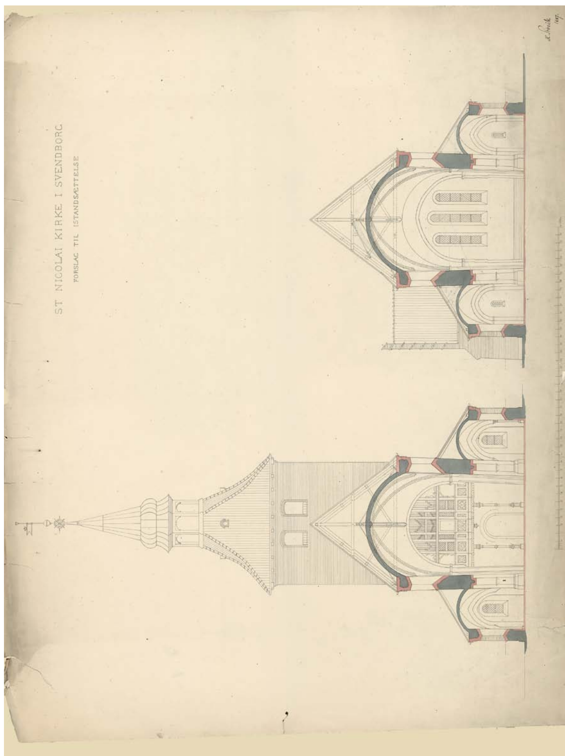
Fig. 18a-b. Tværsnit. 1:300. Forslag til restaurering ved H. B. Storck 1887. a. Set mod vest. b. Set mod øst. – Cross sections. Proposal for restoration by H. B. Storck, 1887. a. Looking west. b. Looking east.
