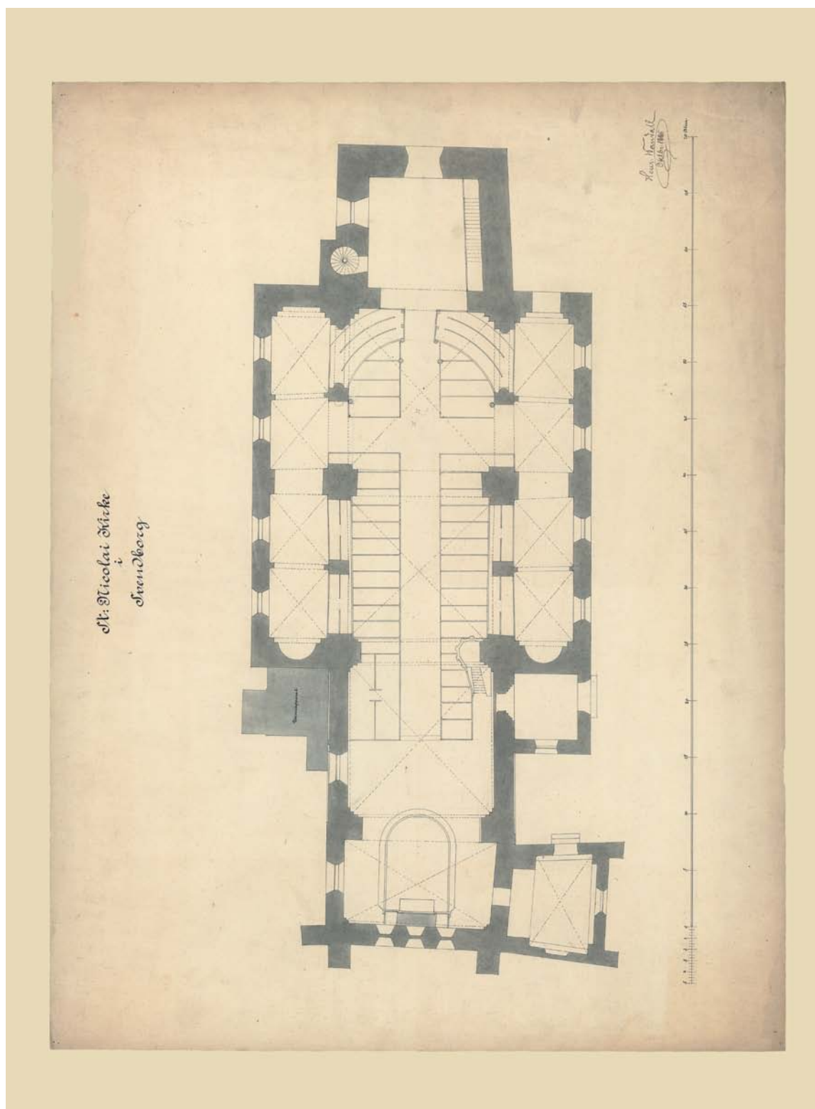
Fig. 10. Grundplan. 1:300. Vest opad. Opmåling ved H. Wandall 1886. — Groundplan. West at top, 1886.
