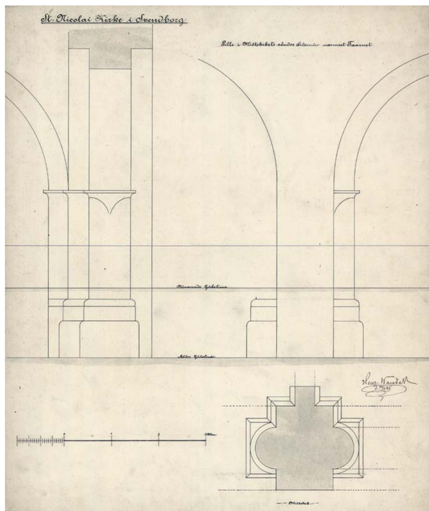
Fig. 56. Pille i midtskibets søndre sidemur nærmest tårnet. 1:50. Opmåling ved H. Wandall 1886. – Pillar close to the tower in the south side-wall of the nave, 1886.
