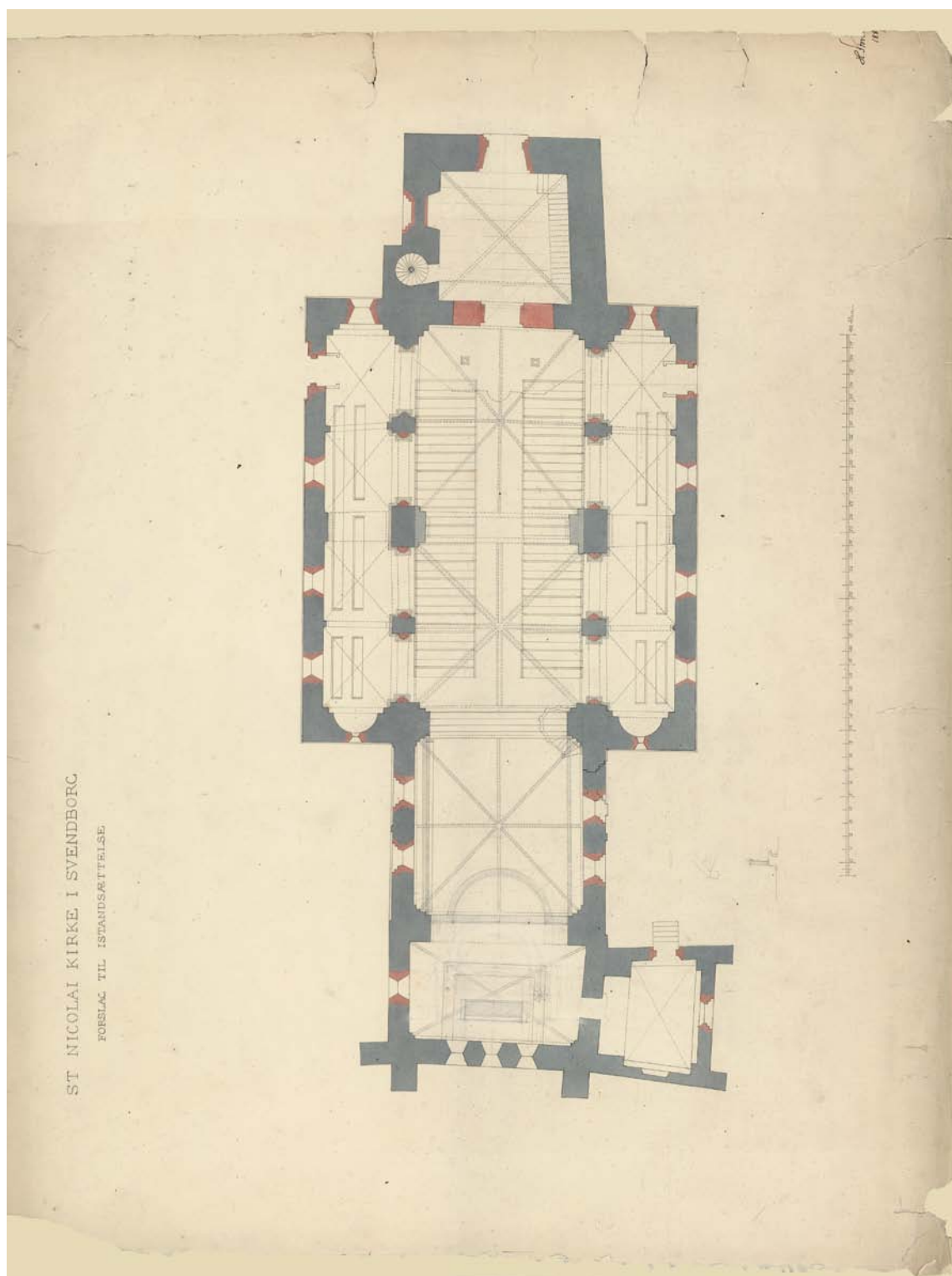
Fig. 16. Grundplan. 1:300. Vest opad. Forslag til restaurering ved H. B. Storck 1887. — Groundplan. West at top. Proposal for restoration by H. B. Storck, 1887.
