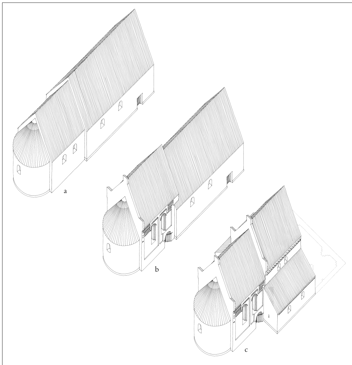
Fig. 28a-c. Aksonometrisk rekonstruktion af stadier i kirkens bygningshistorie 1:500. a. Før 1200. †Romansk kampestenskirke. b. 1200-1225. Senromansk †apsis og kor af teglsten samt ældre skib. c. 1225-1250. Senromansk †apsis og kor samt første fase af basilika. Tegnet af Thomas Bertelsen 2011. — Axonometric reconstruction of phases of the building-history of the church, 1:600. a. Before 1200. †Romanesque granite-built church. b. 1200-1225. Brick-built late Romanesque †apse and chancel, and older nave. c. 1225-1250. Late Romanesque †apse and chancel, and first phase of basilica.
