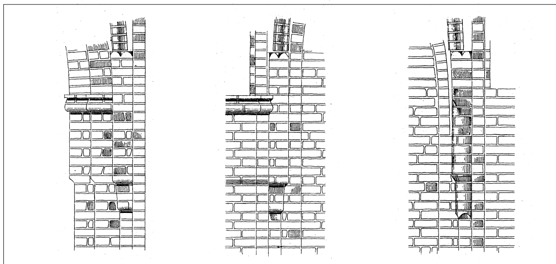
Fig. 53a–c. Senromanske hvælpiller i koret (s. 131). 1:50. a. Nordvestre hjørne set mod vest. b. Nordvestre hjørne set mod nord. c. Nordøstre hjørne set mod nord. Målt og tegnet af Poul Holsøe. – Late Romanesque vault-pillar in the chancel. a. The northwest corner, looking west. b. The northwest corner, looking north. c. The northeast corner, looking north.
