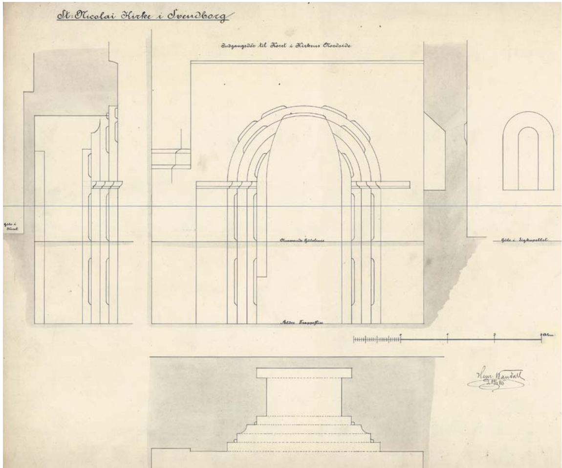
Fig. 45. Opstalt og snit af portal i korets nordside. 1:50. Opmåling ved H. Wandall 1886. – Elevation and cross section of the portal in the north side of the chancel, 1886.
