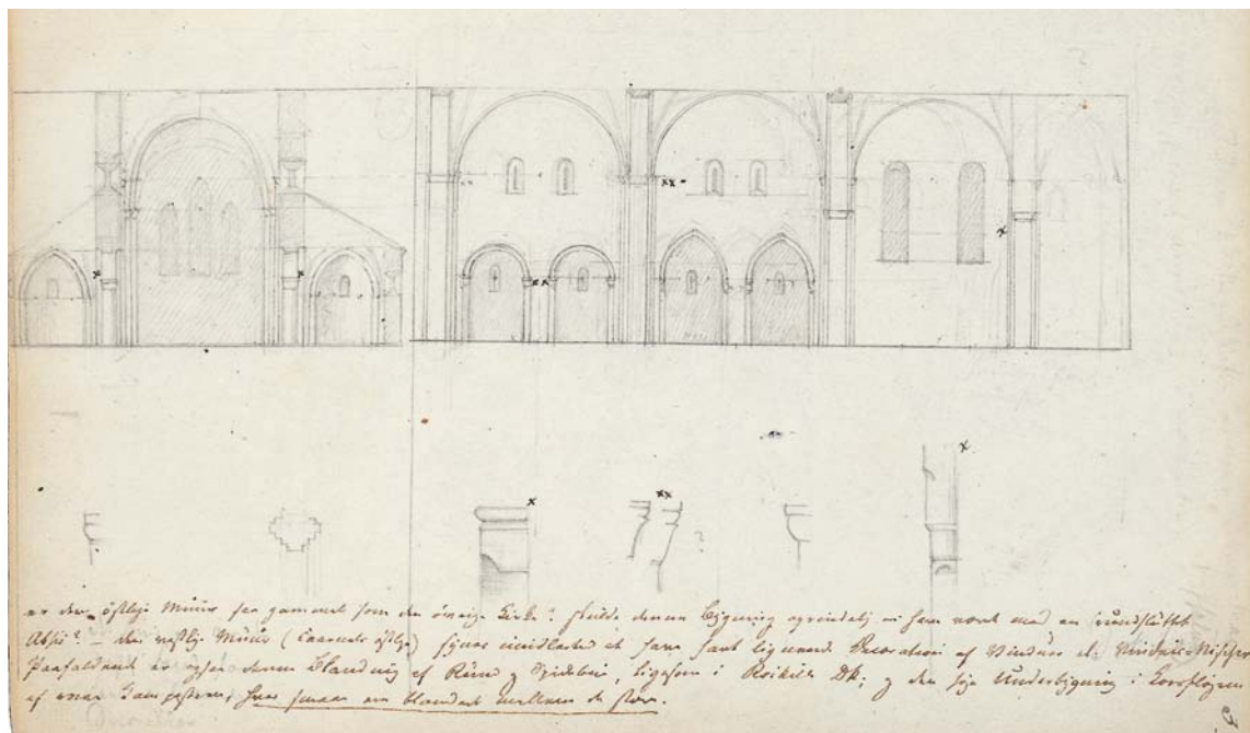
Fig. 7. Tværsnit set mod øst, opstalt af midtskibets, korets og korforlængelsens nordvæg samt diverse detaljer (s. 126). Tegning af N. L. Høyen i notebog 1830. – Cross-section looking east, elevation of the north wall of the nave, the chancel and the chancel extension, with diverse details, 1830.
