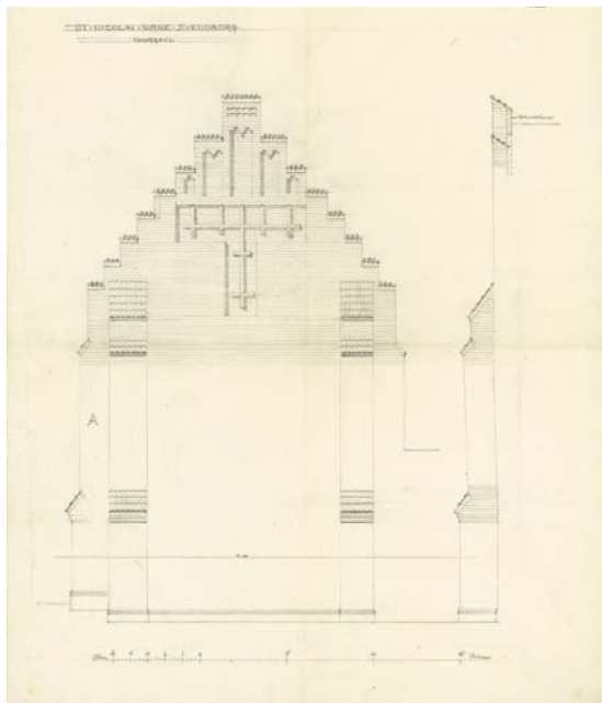
Fig. 73. Korforlængelsens østgavl før restaurering, opstalt og snit mod syd. 1:300. Usigneret opmåling 1892-94. – The east gable of the chancel extension before the restoration, elevation and section looking south. 1:300. Unsigned, 1892-94.
