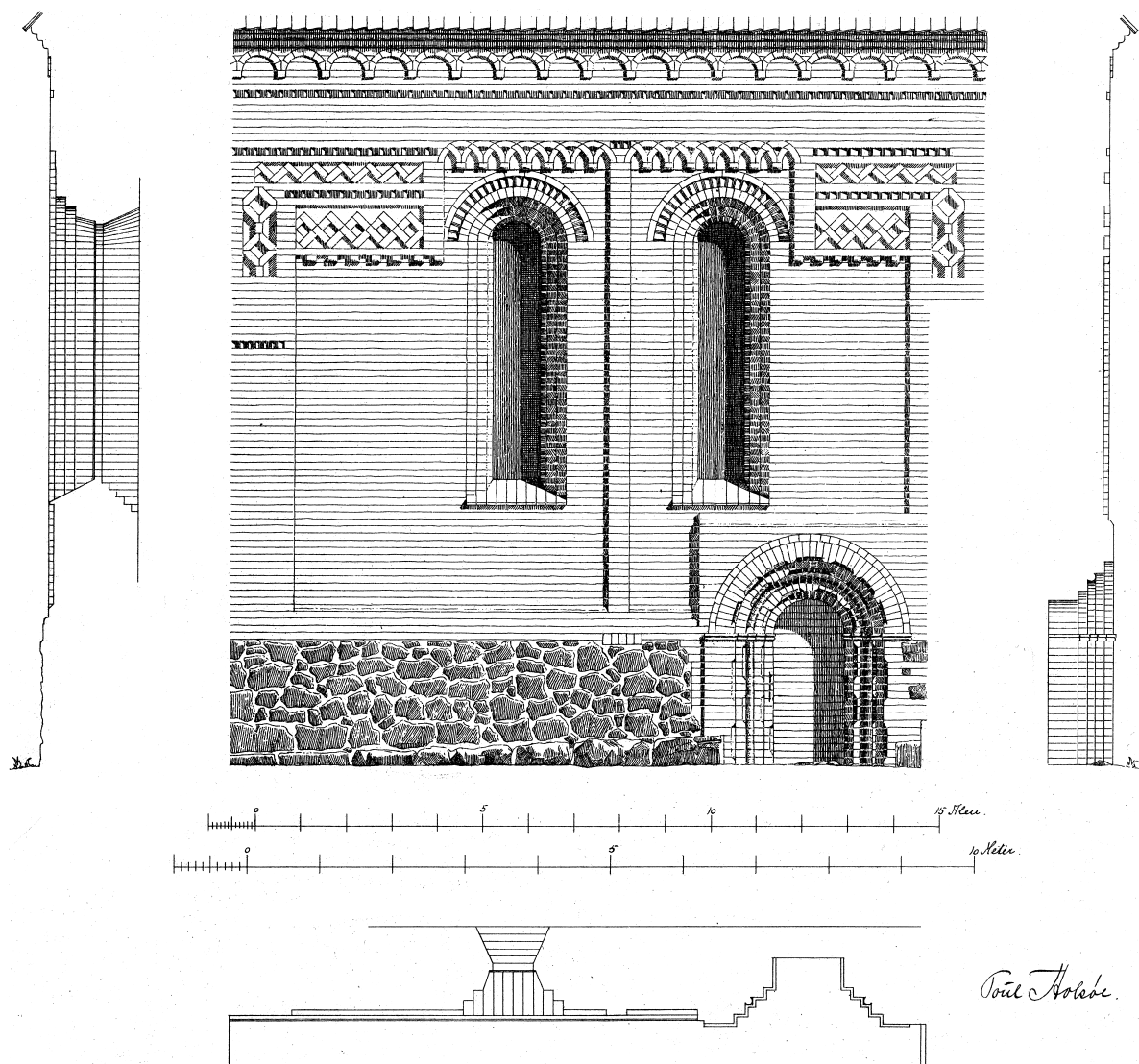
Fig. 30. Korets nordfacade. 1:100. Målt og tegnet af Poul Holsøe 1898. – North facade of the chancel.
