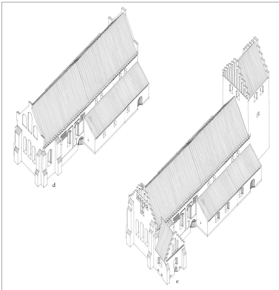
Fig. 28d-e. Aksonometrisk rekonstruktion af stadier i kirkens bygningshistorie 1:500. d. 1225-1250. Senromansk \uparrow apsis og kor samt anden fase af basilika. e. O. 1550. Sakristiet og tårnet er opført. Tegnet af Thomas Bertelsen 2011. – d. 1225-50. Late Romanesque \uparrow apse and chancel, and second phase of basilica. e. c.1550. The vestry and the tower have been built.
