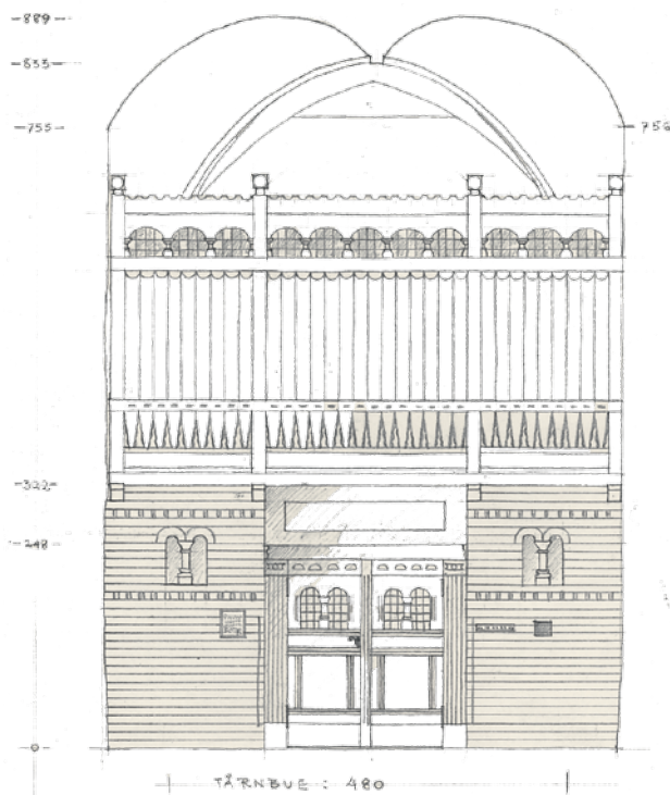
Fig. 114. Bagsiden af \dagger orgel nr. 4 (s. 205). 1:100. Tegning af I. Arthur-Nielsen. – Back of \dagger organ no. 4. Drawing by I. Arthur-Nielsen.
