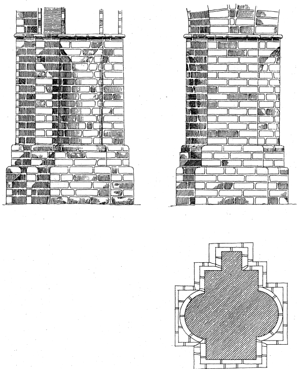
Fig. 58. Arkadepille i nordsiden af midtskibets 2. fag. 1:50. Målt og tegnet af Poul Holsøe. – Pillar in the second bay of the arcade on the north side of the nave.
