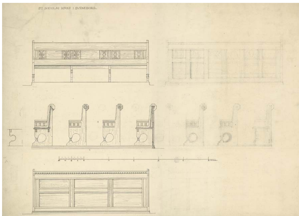
Fig. 105. Forslag til stolestader, 1892-94 (s. 194). 1:50. Tegning af H. B. Storck. – Proposal for pews, 1892-94. Drawing by H. B. Storck
