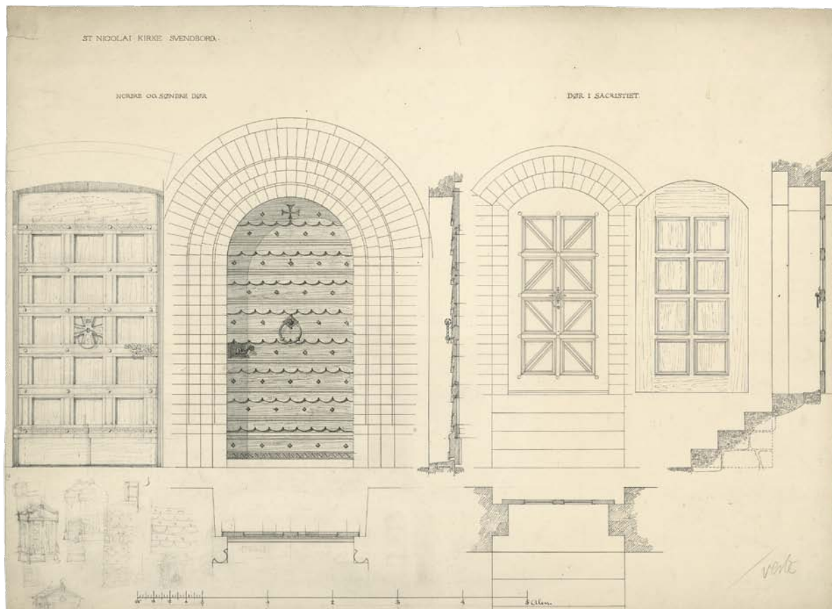
Fig. 110. Forslag til udvendige dørfløje nr. 1-3, 1892-94 (s. 201). Nr. 1 (th.) i sakristiet, nr. 2-3 (tv.) i sideskibene. 1:50. Tegning af H. B. Storck. – Proposal for outer doors, nos. 1-3, 1892-94. No. 1 in the vestry (right) and nos. 2-3 in the aisles (left). Drawing by H. B. Storck.
