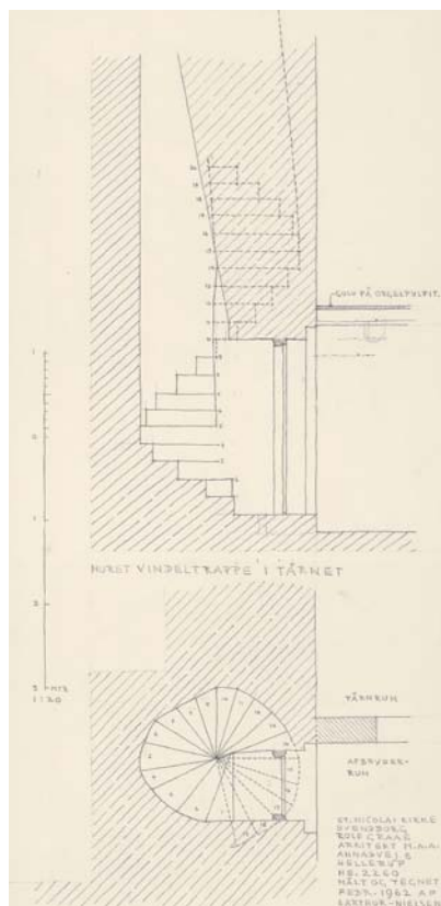
Fig. 69. Trappe til første mellemstokværk i tårnet (s. 151). 1:100. Opmåling ved I. Arthur-Nielsen 1962. – Staircase to the first landing in the tower.
