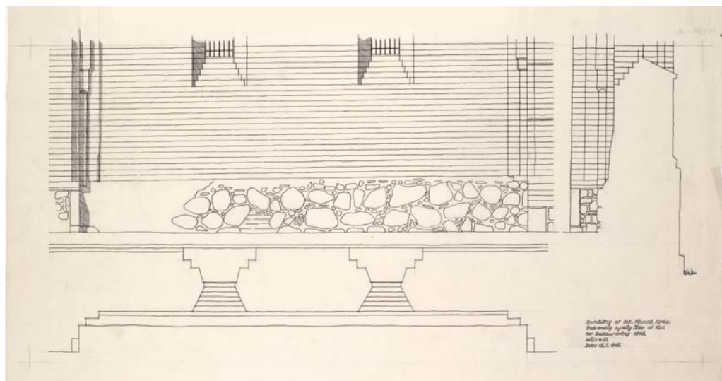
Fig. 27. Opstalt af den nederste del af korets sydvæg. 1:100. Kampestensmurværket forinden er fra den ældre tækirke. Opmåling ved A. Jensen 1949. Danmarks Kunsthbibliotek. – Drawing of the lower part of the chancel's south side (interior), 1949. The boulders are from earlier tækirch.
