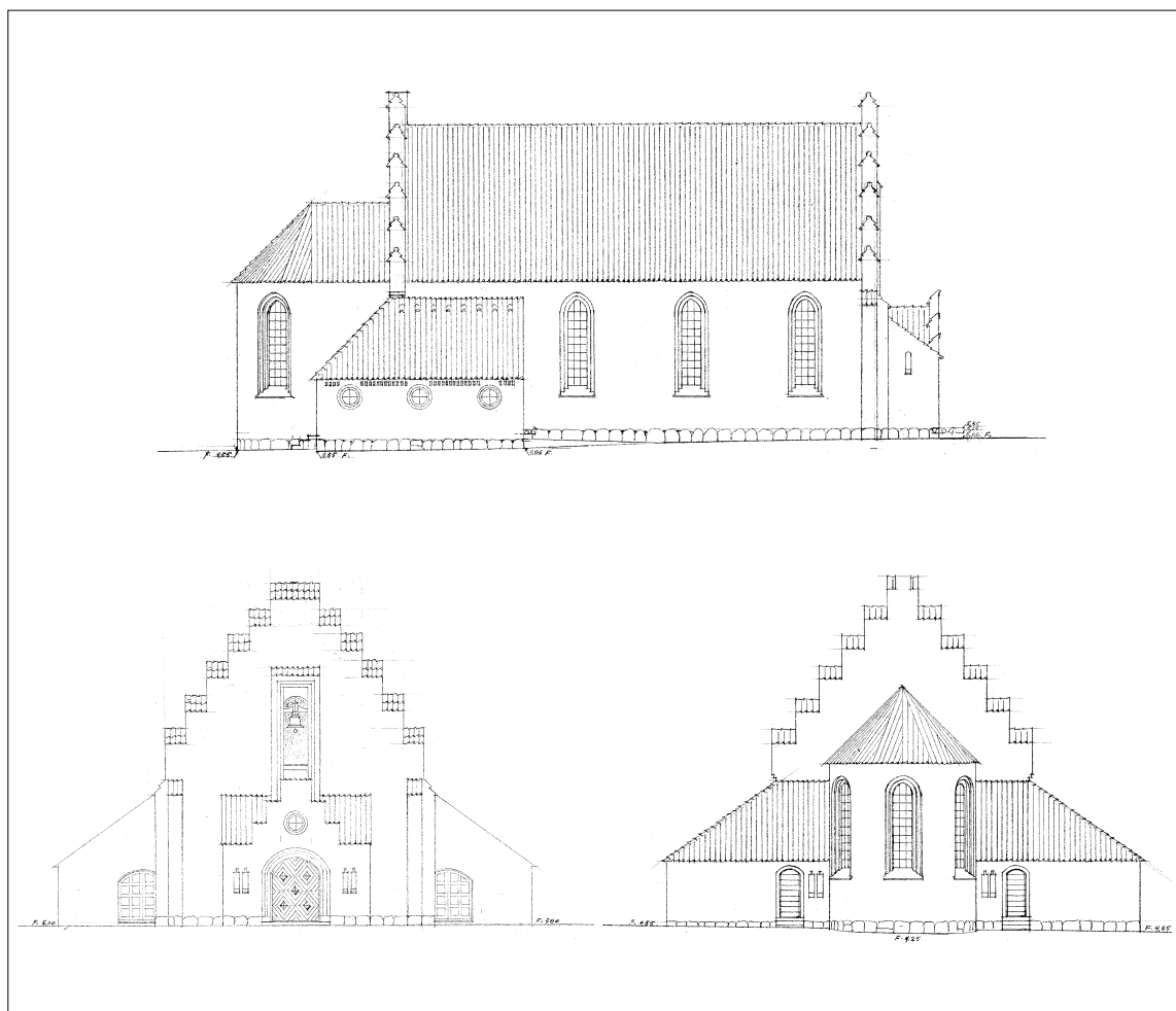
Fig. 4. Forslag til kapel på Svendborg Nye Kirkegård. Opstalter set fra vest, syd og nord, tegnet af Andreas Jensen 1931. 1:300. Tegninger i Danmarks Kunstmuseum. – Proposal for a chapel at Svendborg Nye Kirkegård. Elevations seen from the west, south and north.
