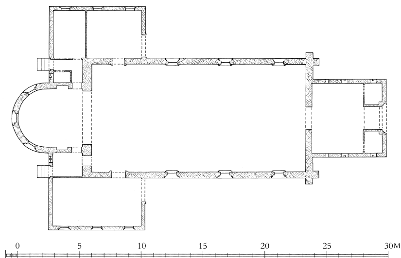
Fig. 3. Grundplan 1:300. Tegnet af Merete Rude 2012 efter Andreas Jensen 1931, suppleret af Ebbe Lehn Petersen 1978. Øst opad. – Ground plan. East up.
